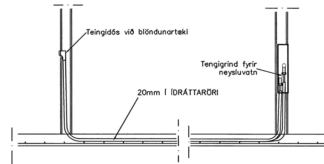
TENING NEYSLUVATNSLAGNA 1:20
