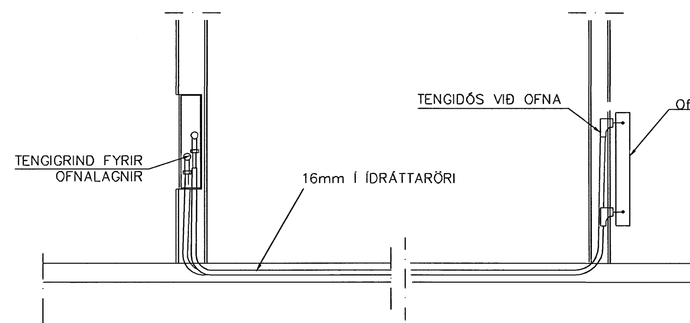
TENING OFNALAGNALAGNA 1:20
