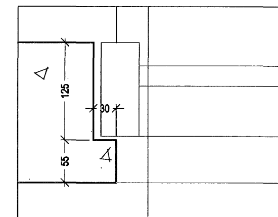
MÁLSETNING Í KRINGUM GLUGGAOP ATH. MÁL Í KRINGUM GÓLFSÍÐA GLUGGA ÞARF AD SAMRÆMA VIÐ ENDANLEGAR GLUGGATEIKNINGAR
