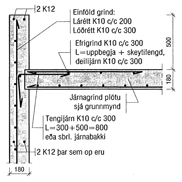
Mkv. 1:20 P1 B08/B09
