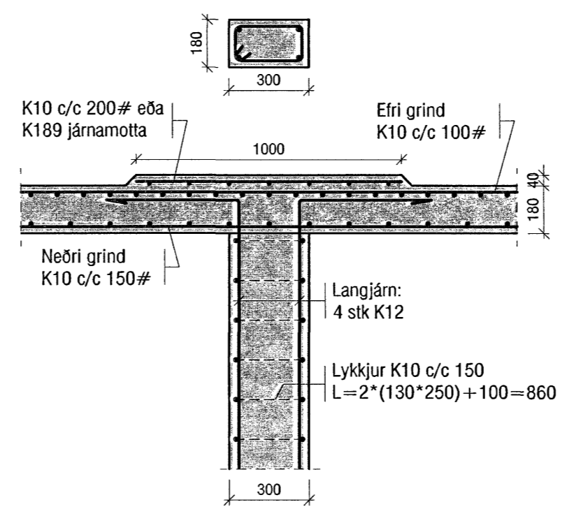
Mkv. 1:20 P7 B08/B09
