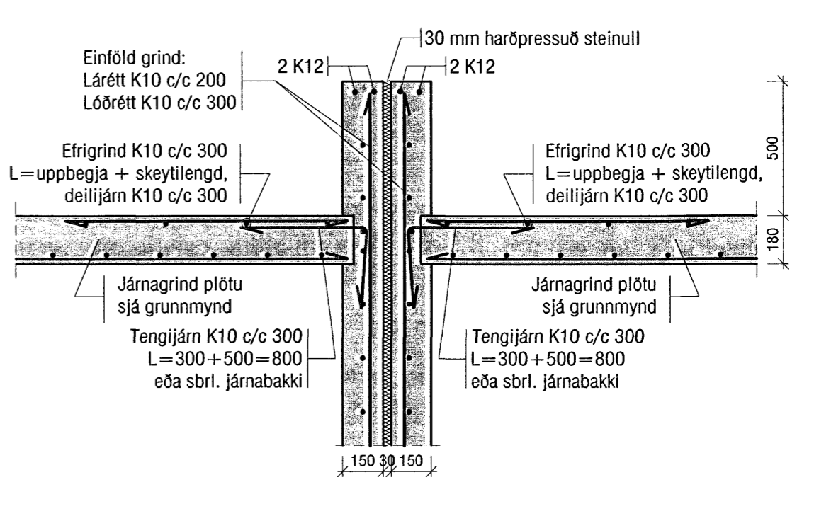
Mkv. 1:20 P8 B08/B09
