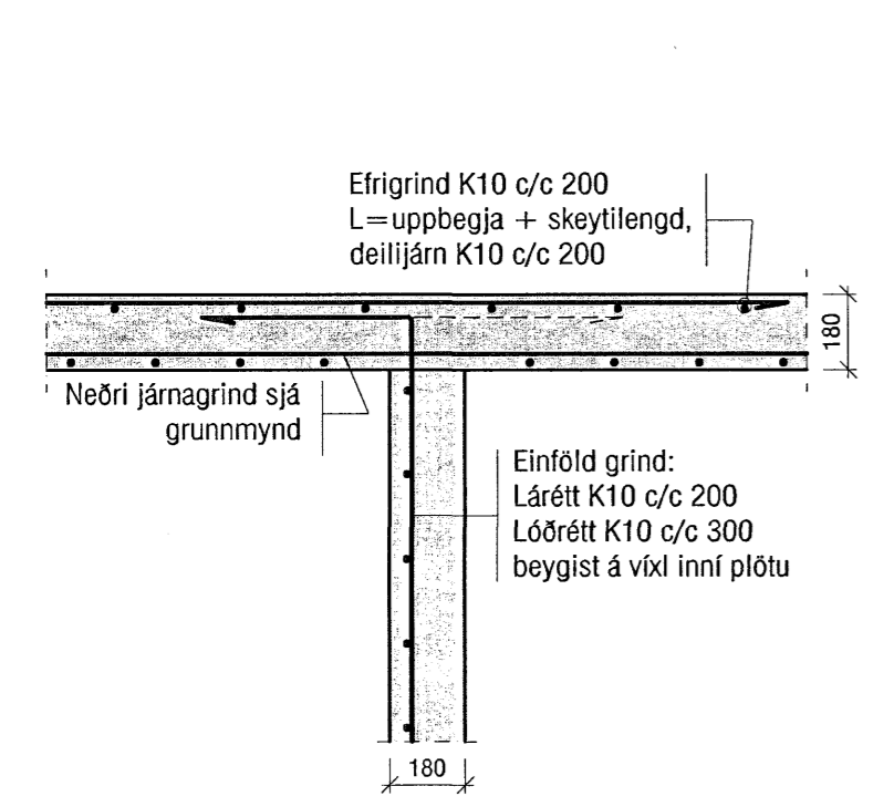
Mkv. 1:20 P5 B08/B09
