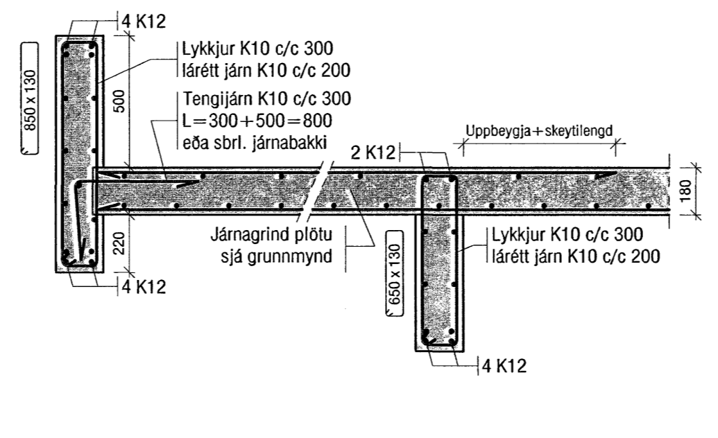
Mkv. 1:20 P3 B08/B09
