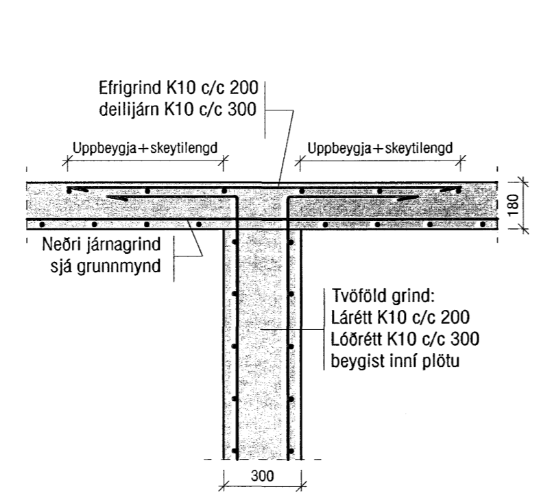
Mkv. 1:20 P6 B08/B09
