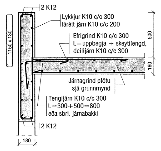
Mkv. 1:20 P2 B08/B09
