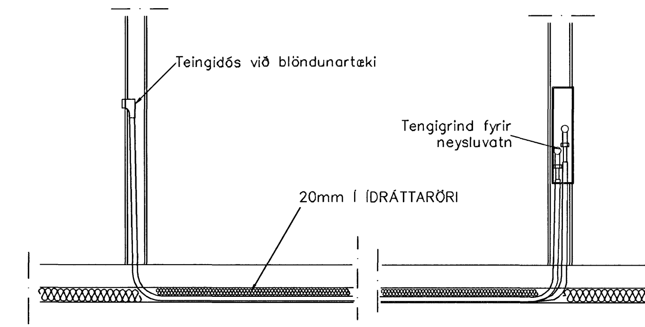
TENING NEYSLUVATNSLAGNA 1:20
