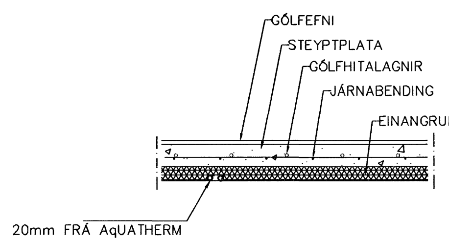
LAGNIR, SNIÐ, 1:20
