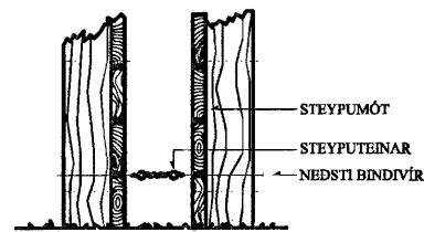
FRÁGANUR Á SAMTENINGUM STEYPUVEINA FYRIR SÖKKULJARÐSKAUT
