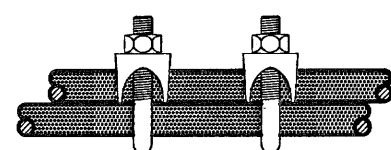
FRÁGANUR Á SAMTENINGUM STEYPUVEINA FYRIR SÖKKULJARÐSKAUT
