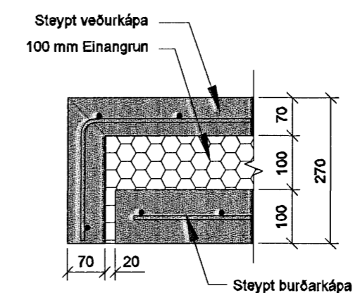
I-105 SNIÐ. 1:10
