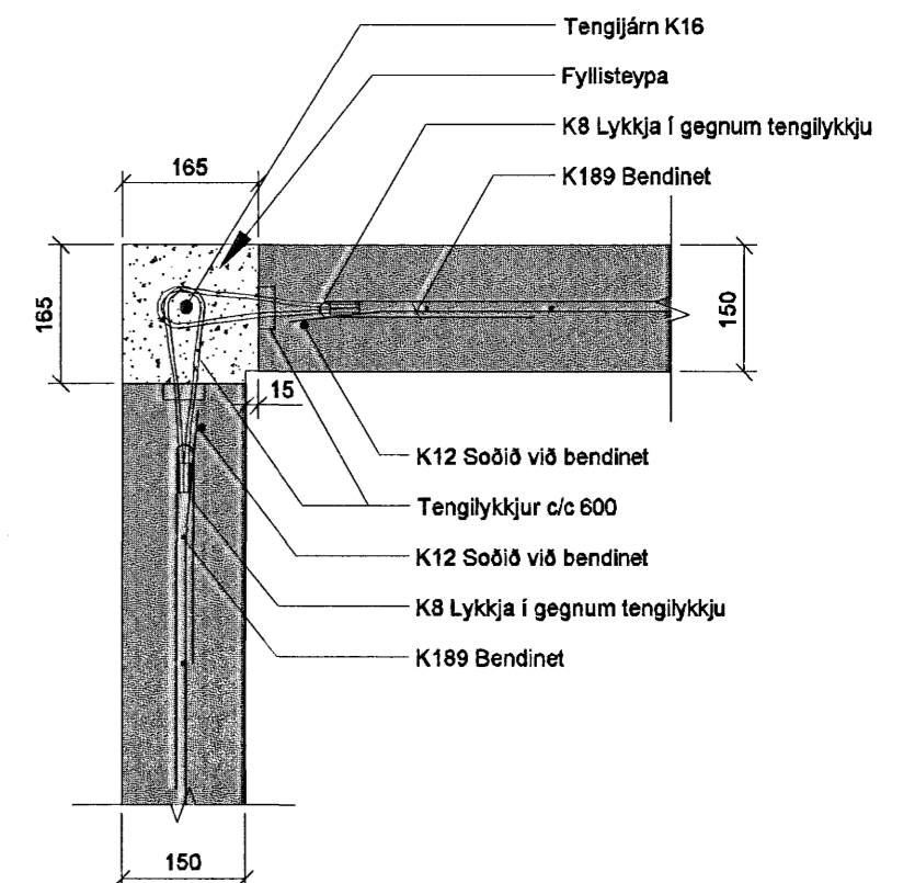
G-105 SNIÐ. 1:10
