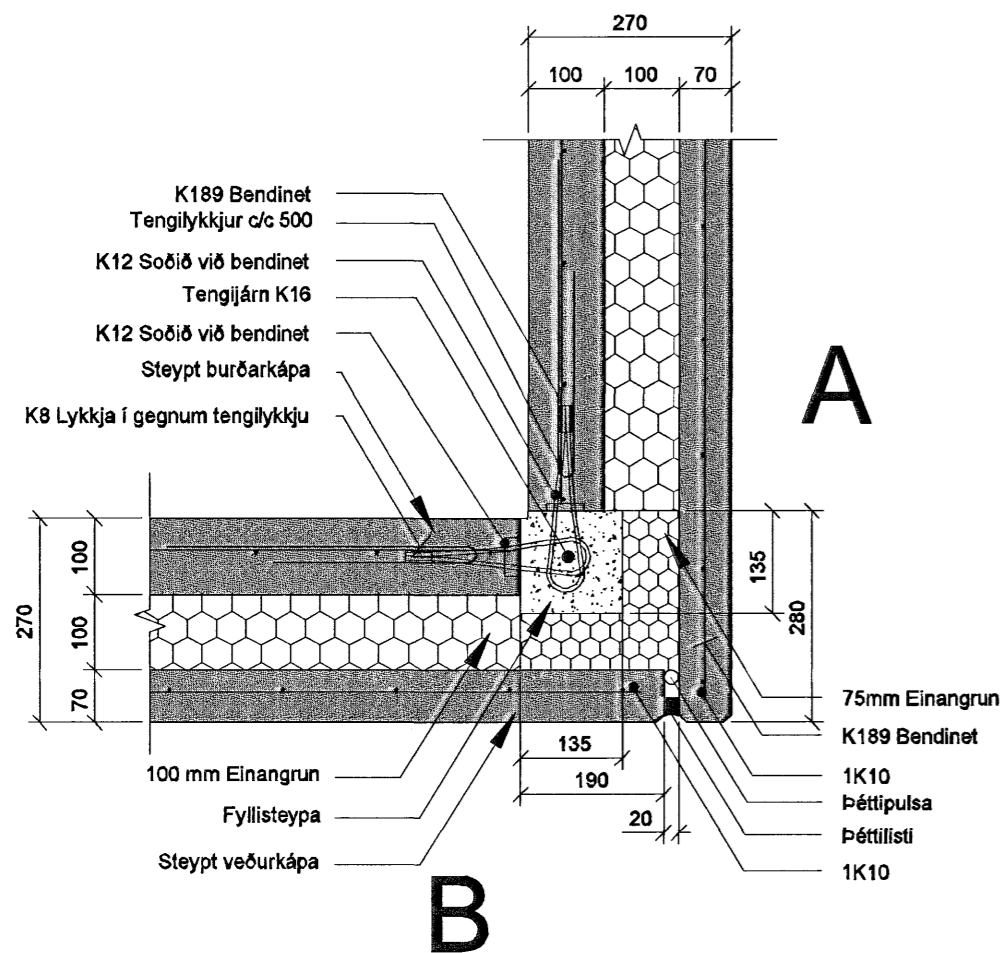
A-105 - úthorn SNIÐ. 1:10
