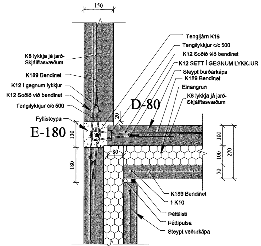
F-105 SNIÐ. 1:10
