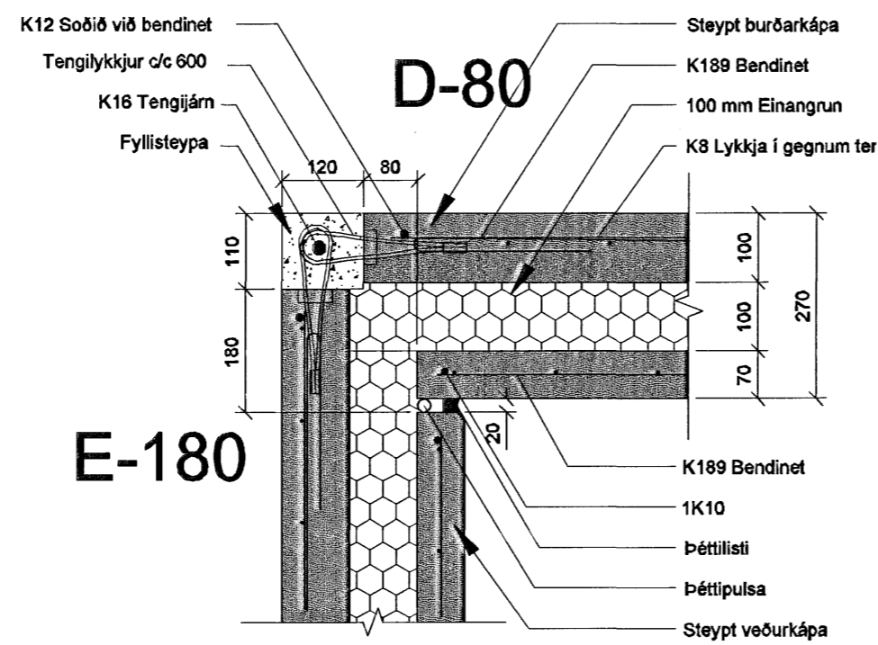
B-105 - Innhorn SNIÐ. 1:10
