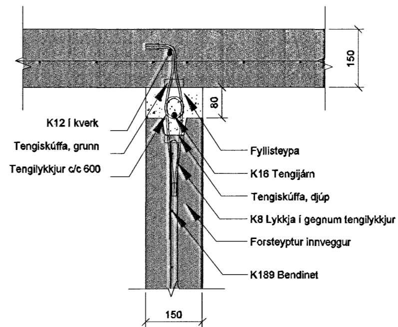
F-105 SNIÐ. 1:10
