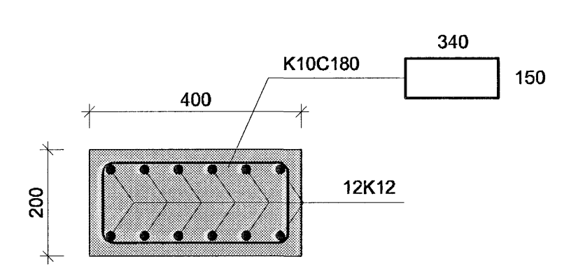
B SNID B-B 04 Mkv. 1/10
