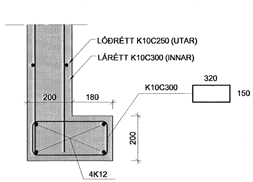
A SNID A-A 04 Mkv. 1/10
