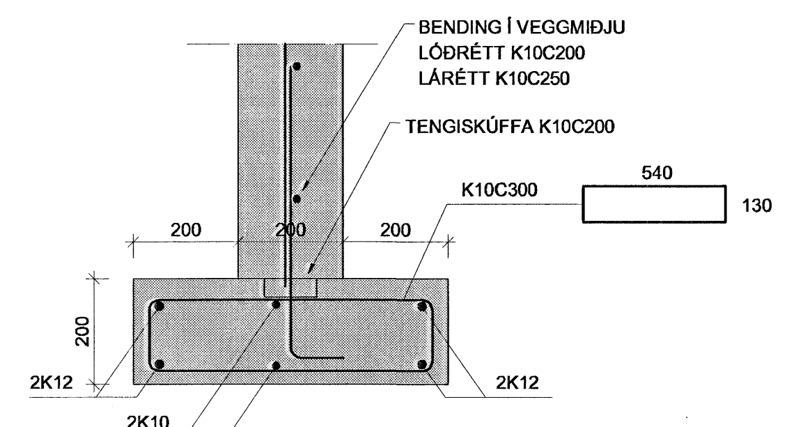
D SNID D-D 04 Mkv. 1/10
