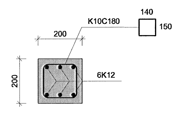
C SNID C-C 04 Mkv. 1/10
