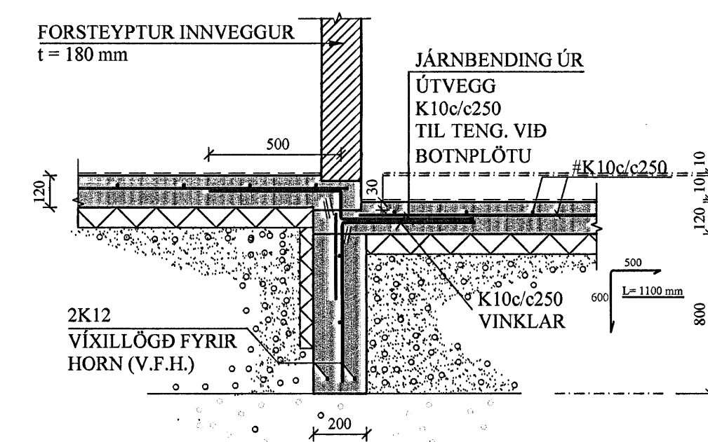
D2 SNIB. 1:20
