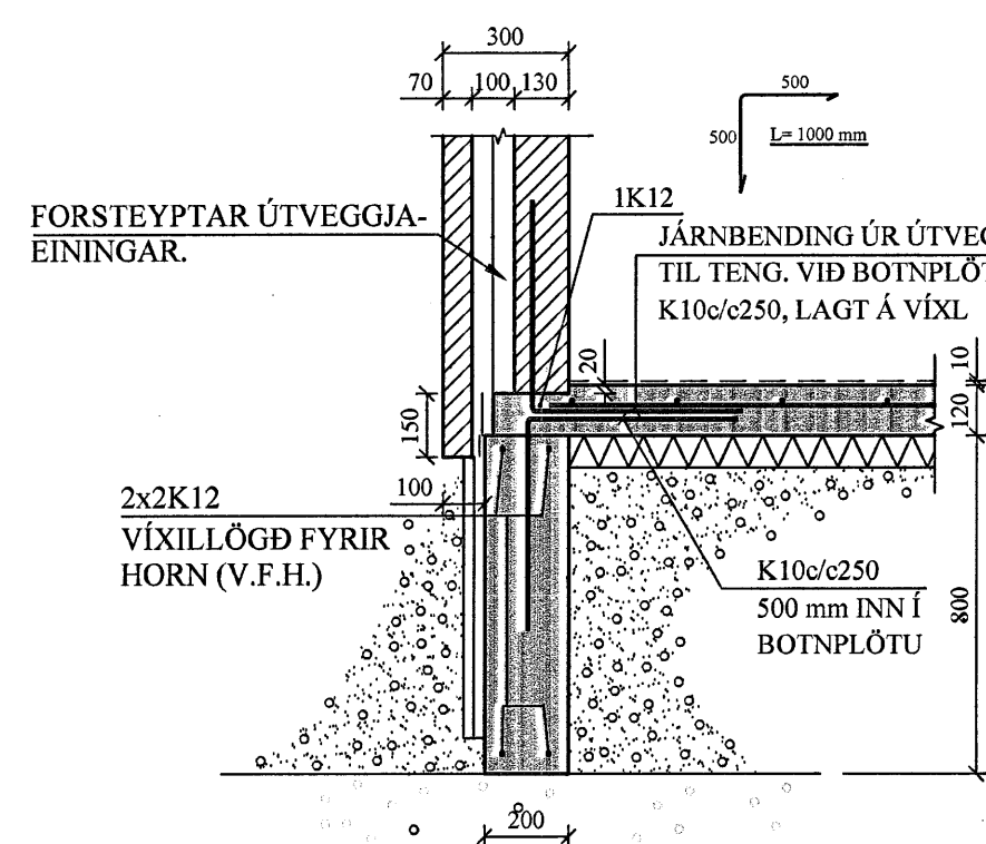
A2 SNIB. 1:20
