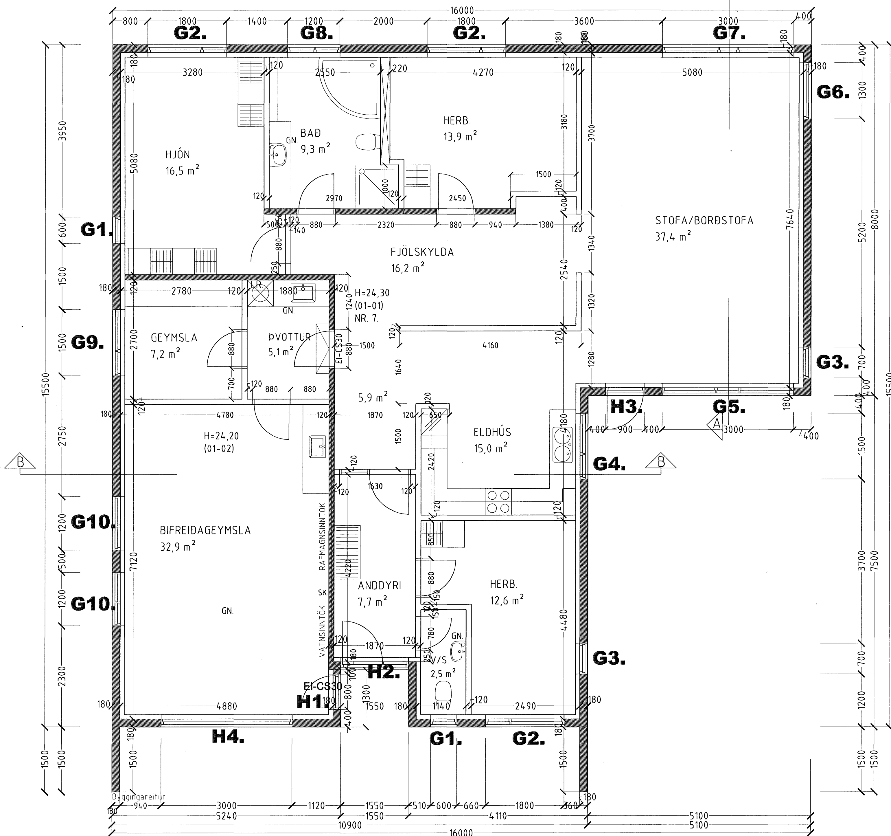
GRUNNMYND 1. HÆÐ MKV. 1:50.
