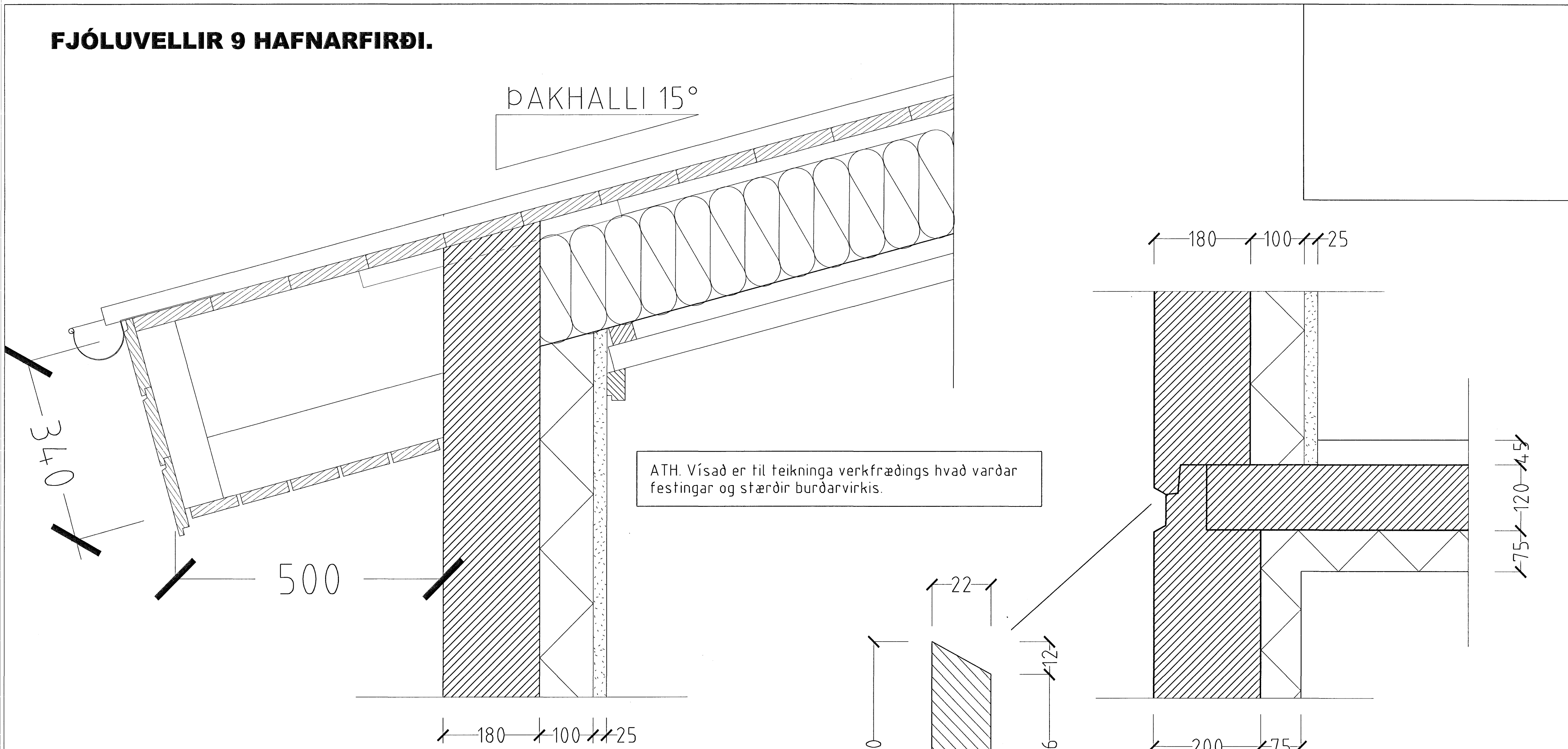
HLUTAMYND ÞAKKANTUR MKV. 1:5.
