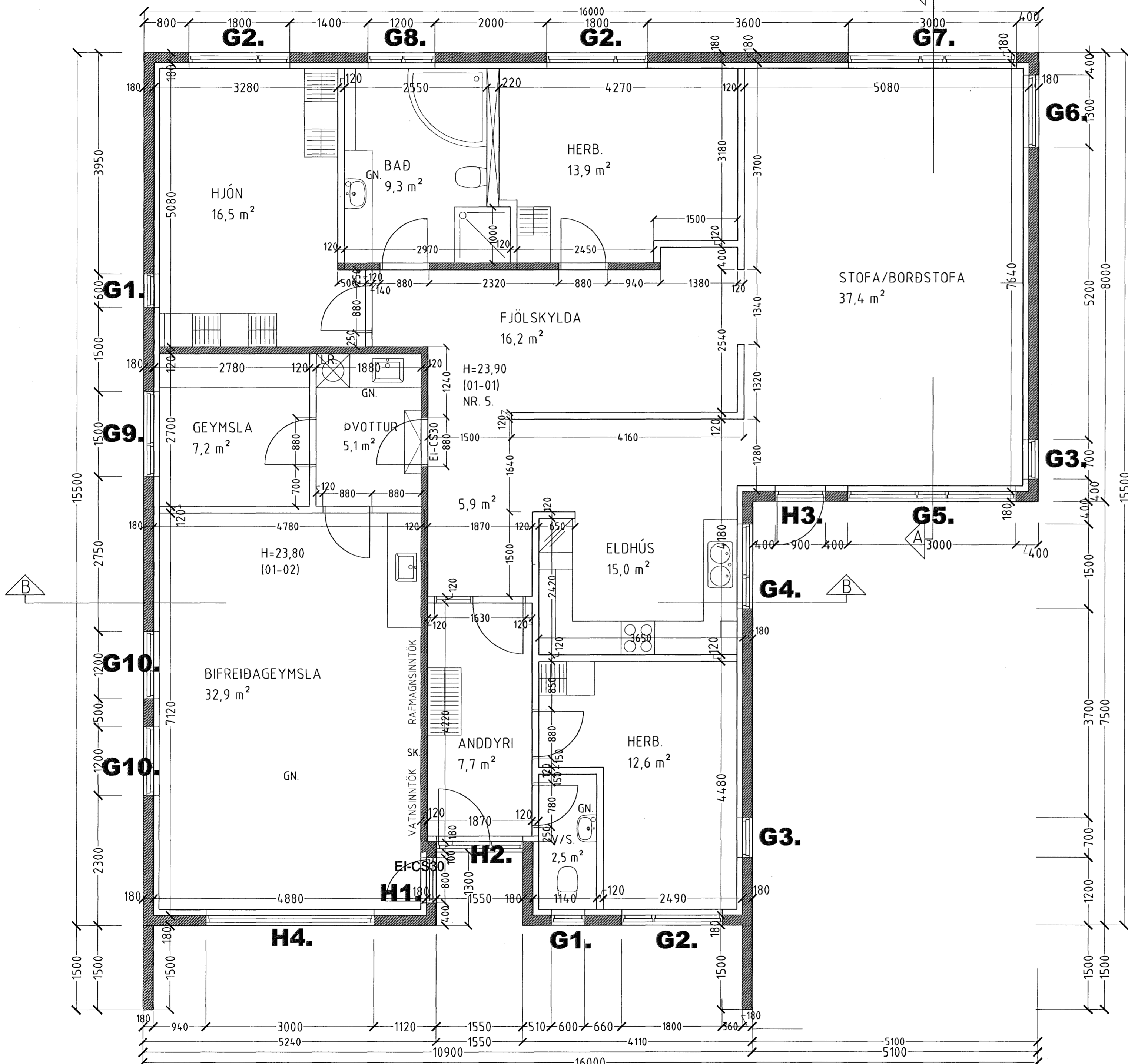
GRUNNMYND 1. HÆÐ MKV. 1:50.
