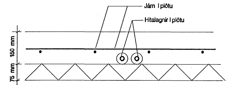
Pversnid í gólfplötu Mkv. 1:10
