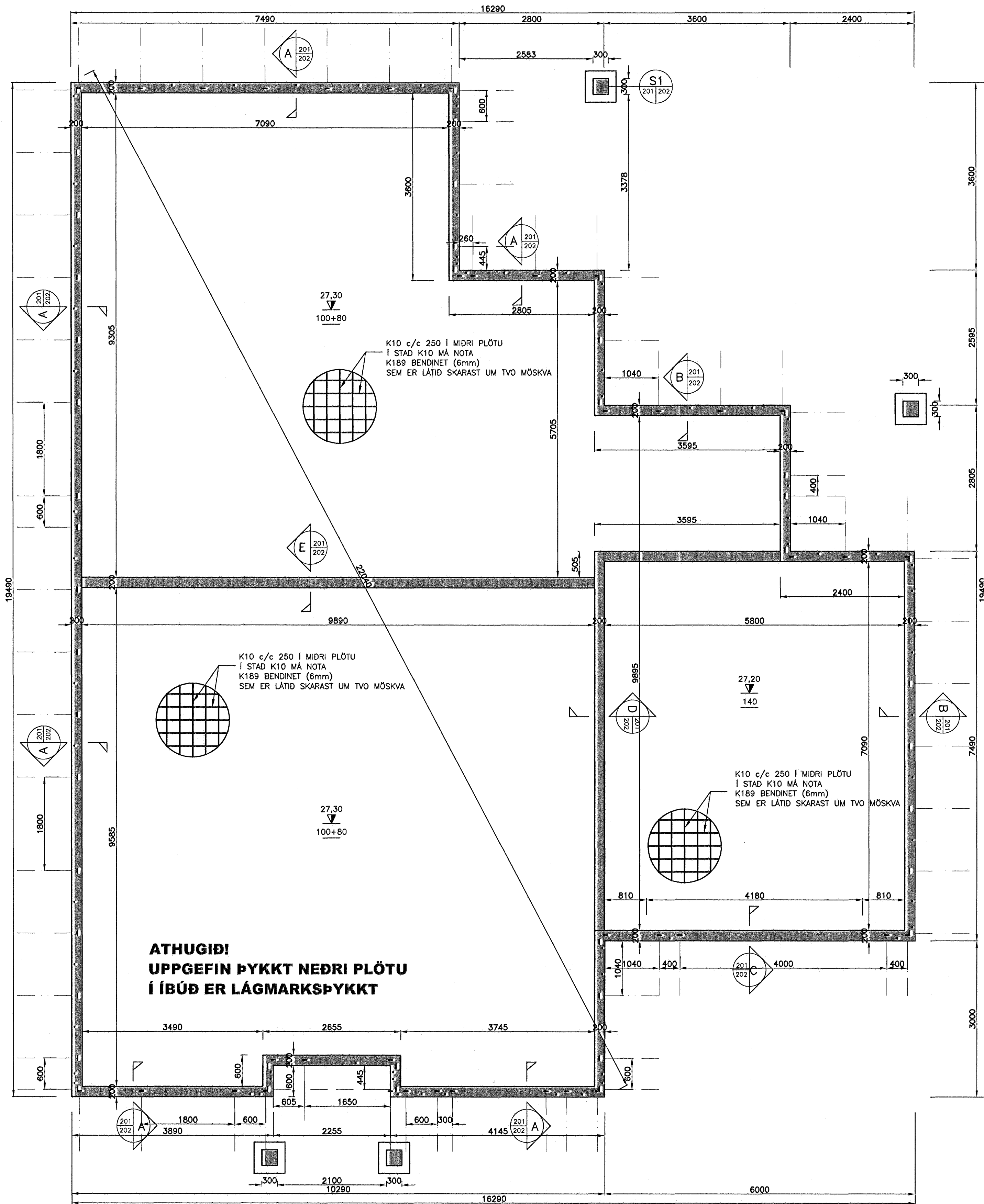
VEGGJAPLAN MKV. 1:50
