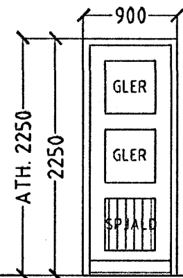
1. STK. BÍLAKJALLARI. HURÐ OPNAST VINSTRI INN.
