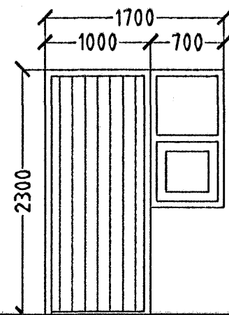
1. STK. HJÓL OG VAGNAR. HURÐ OPNAST HÆGRI INN.
