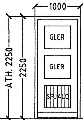
1. STK. HJÓL OG VAGNAR. HURÐ OPNAST VINSTRI INN.
