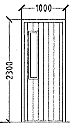
1. STK. STIGAHÚS. HURÐ OPNAST HÆGRI ÚT.
