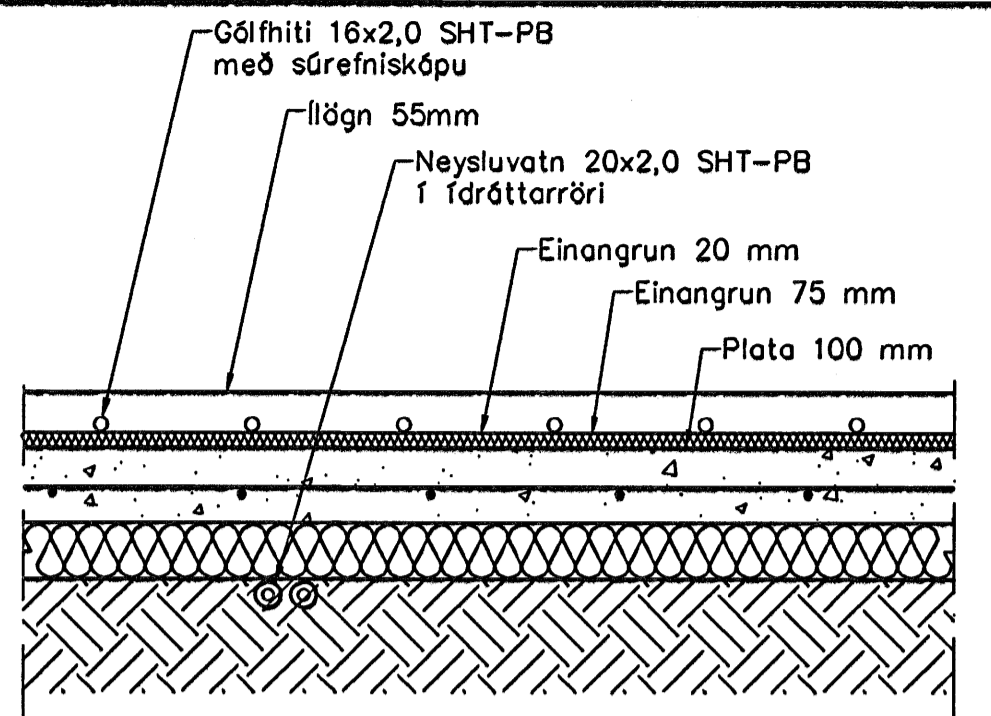
Hita- og vatnslagnir, Sníð í botnplötu, 1:10
