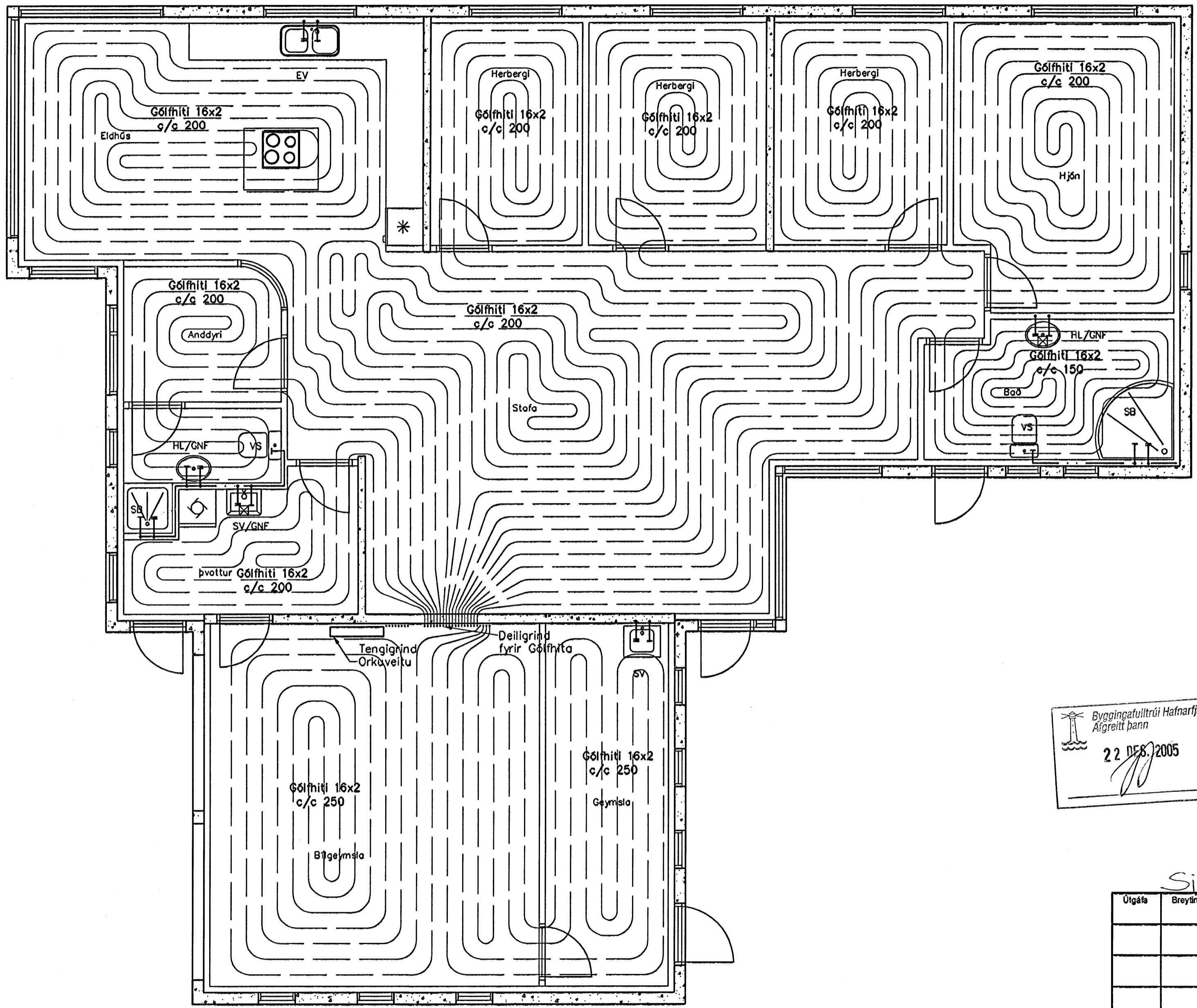
Gólfhitalagnir 1:50
