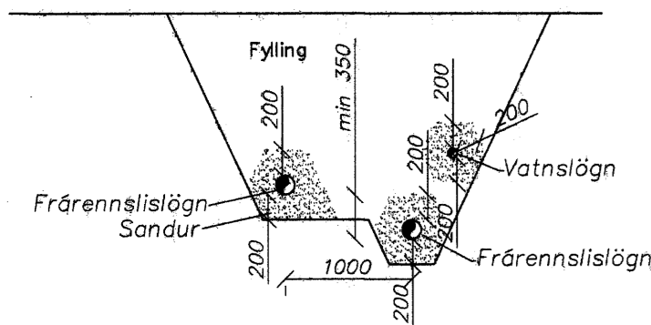
Lagnir í skurði Tvar eða fleiri lagnir í skurði
