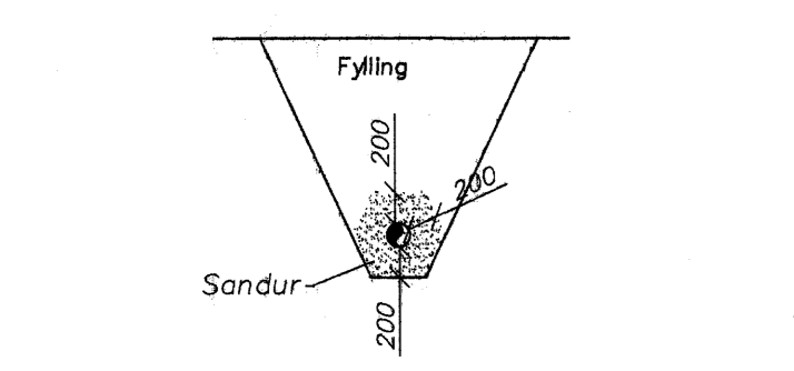
Lagnir í skurði Ein lögn í skurði
