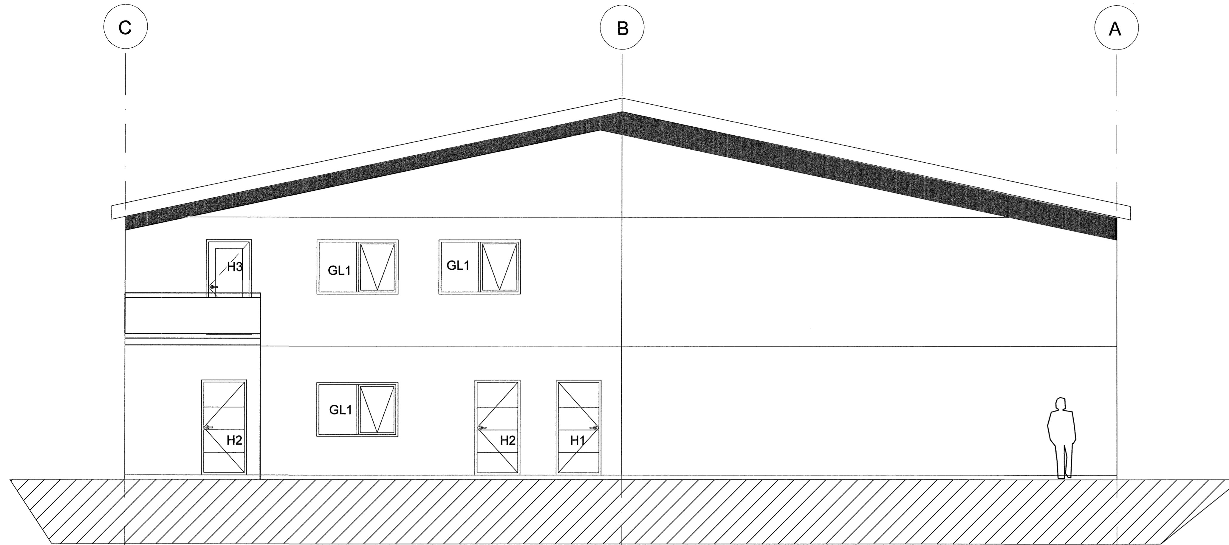
NORÐURHLIÐ, 1:100
