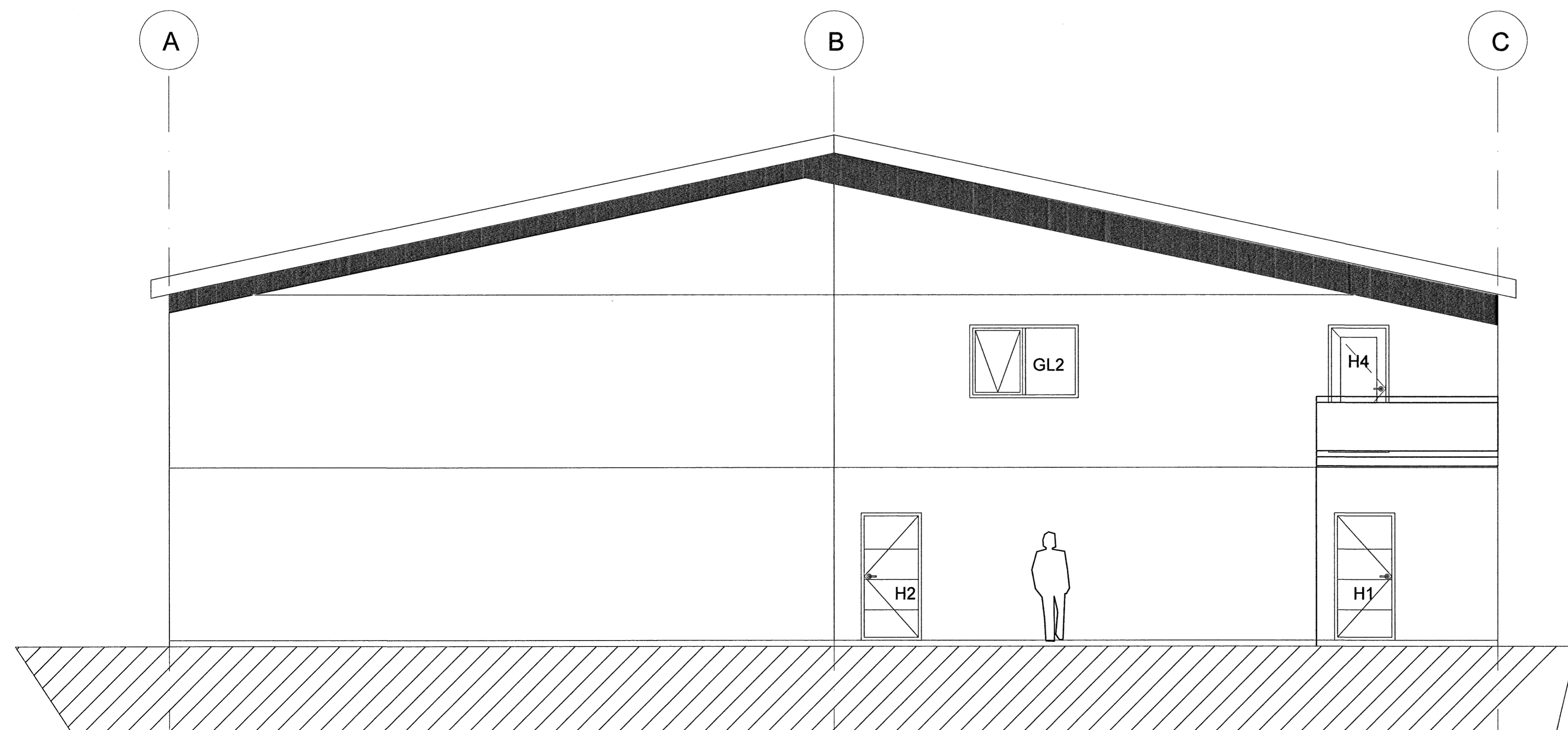
SUÐURHLIÐ, 1:100
