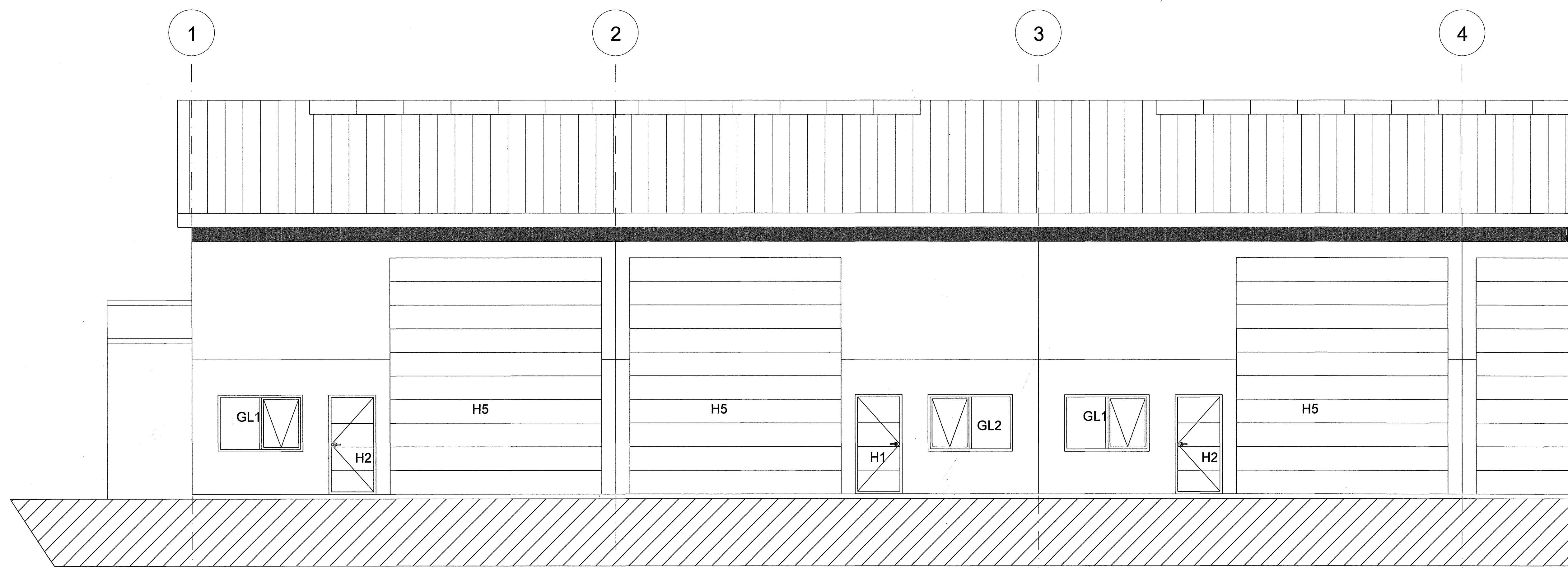
VESTURHLIÐ, 1:100
