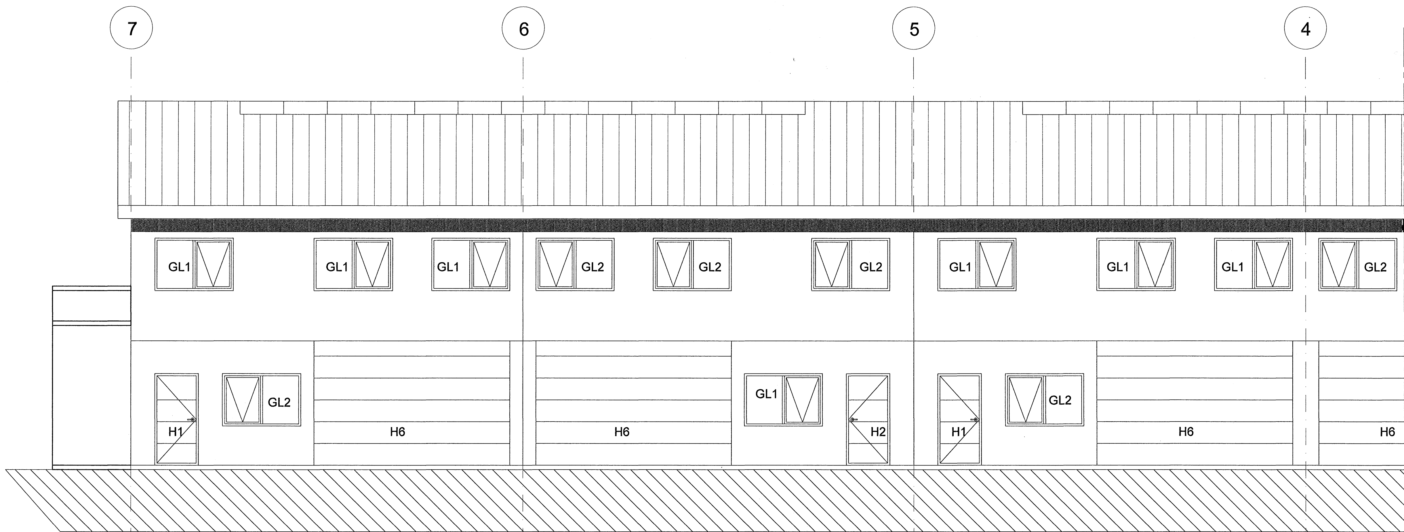
AUSTURHLIÐ, 1:100
