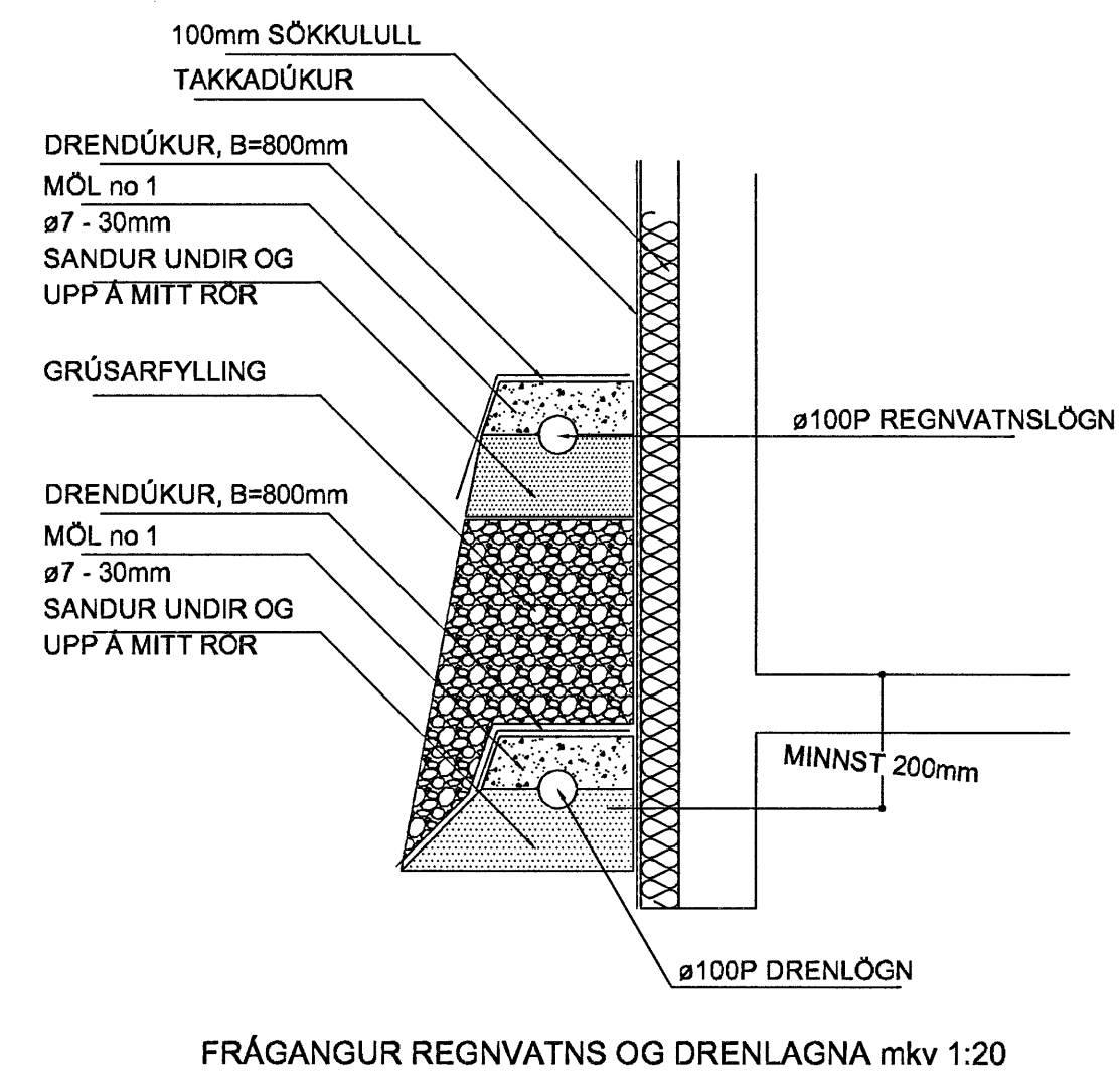
FRÁGANGUR REGNVATNS OG DRENLAGNA mkv 1:20
