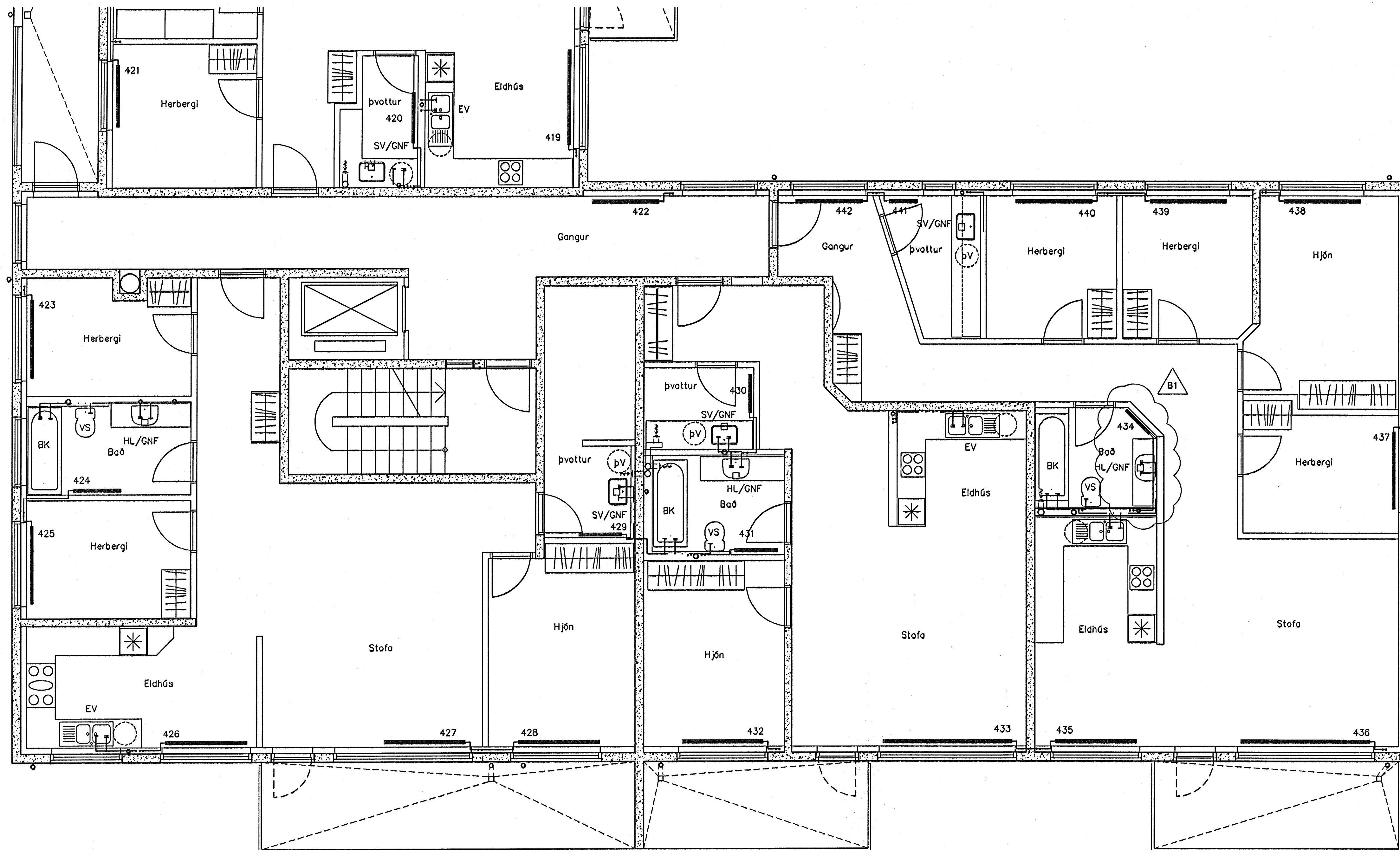
Lagnir 4. Hæð, Grunnmynd, 1:50
