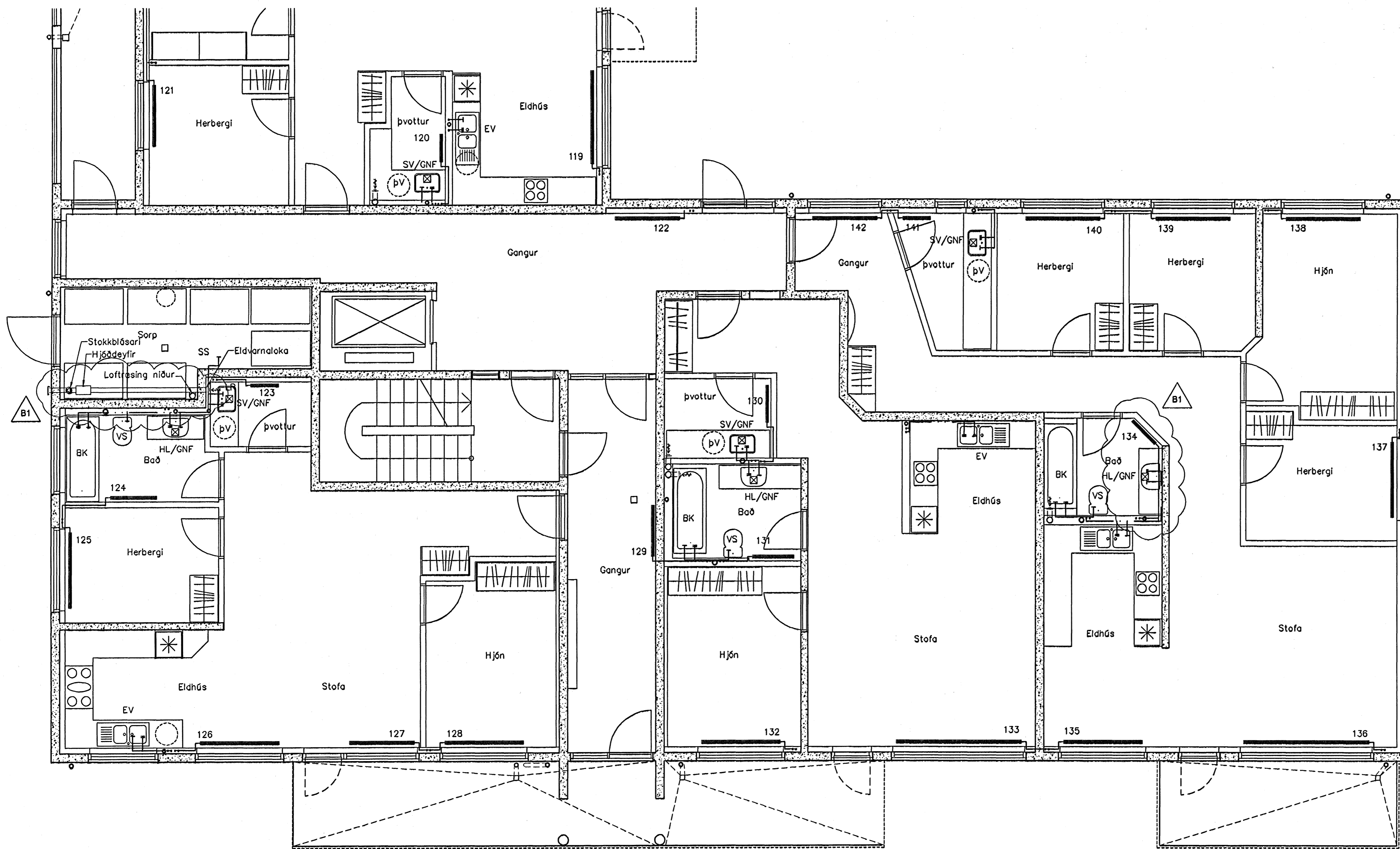
Lagnir 1. Hæð, Grunnmynd, 1:50
