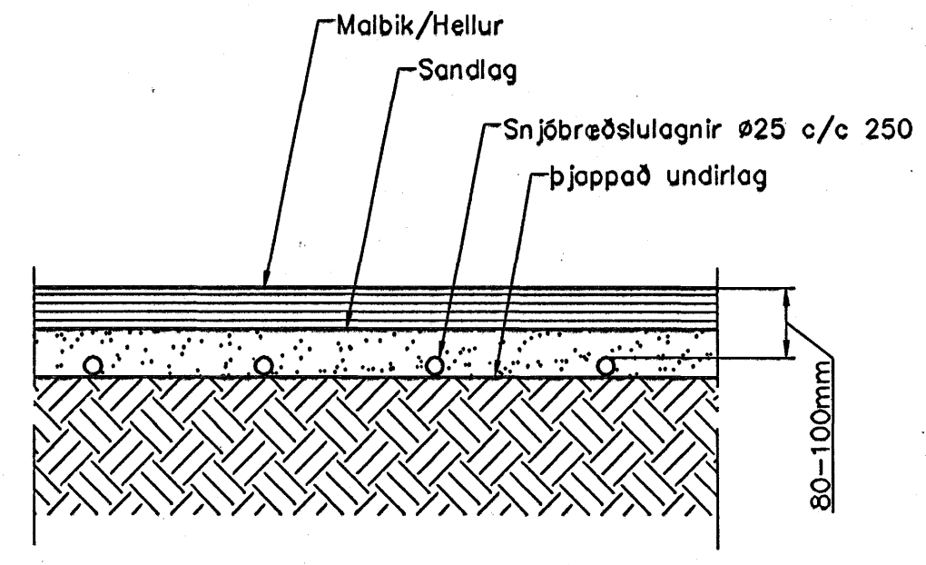
Snjóbræðslulagnir, Sníð, 1:10
