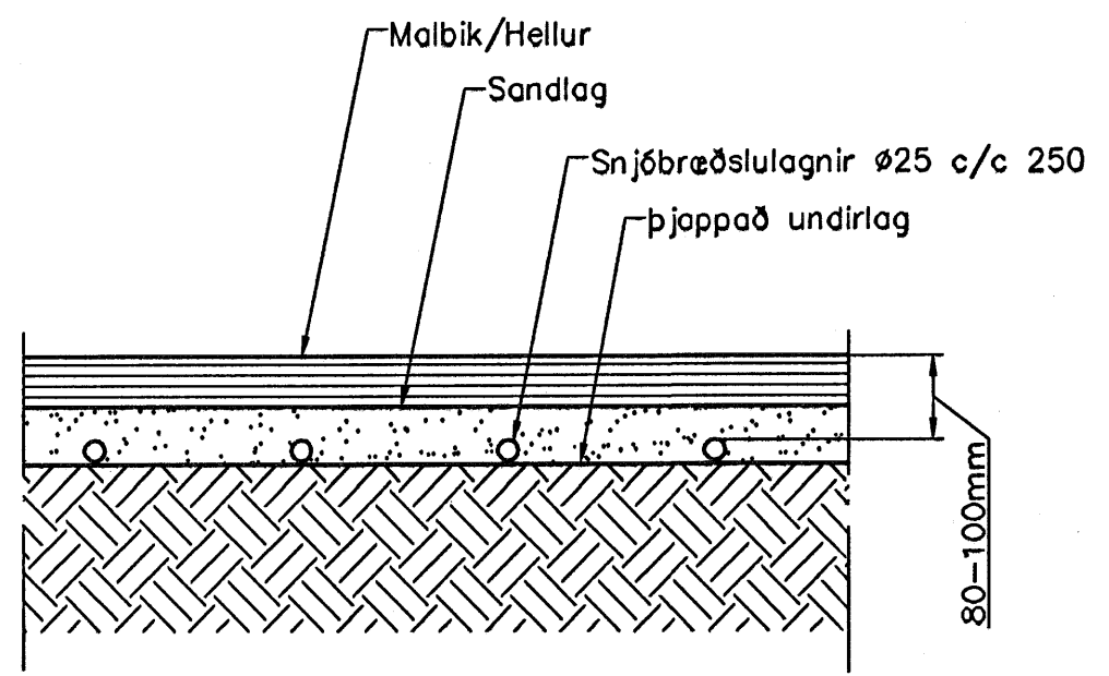
Snjóbræðslulagnir, Snið, 1:10
