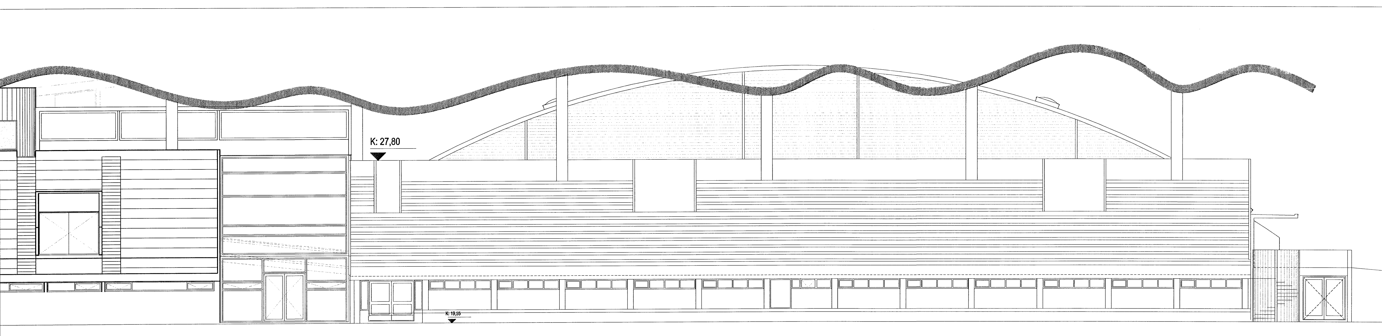
NORÐURHLIÐ D OG A-BYGGINGAR í mkv. 1:100
