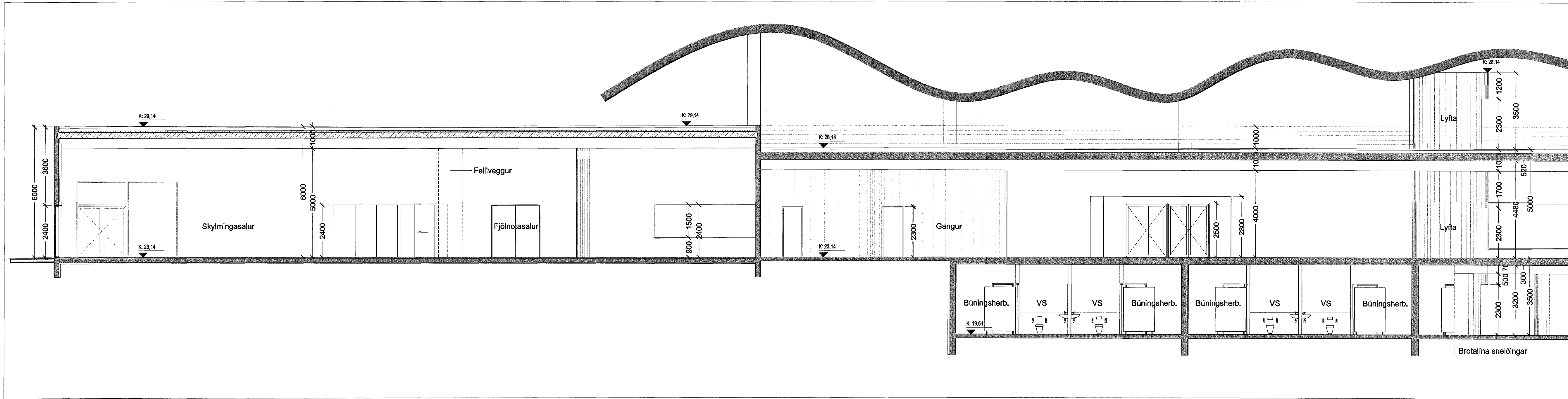
SNID B-B í mkv. 1:100
