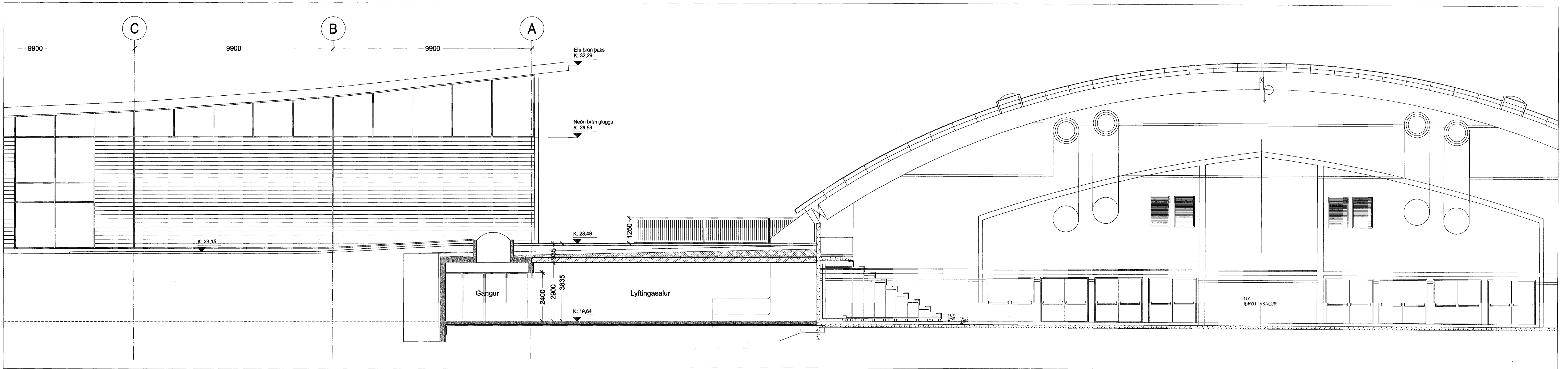
NORÐURHLIÐ E-BYGGINGAR í mkv. 1:100
