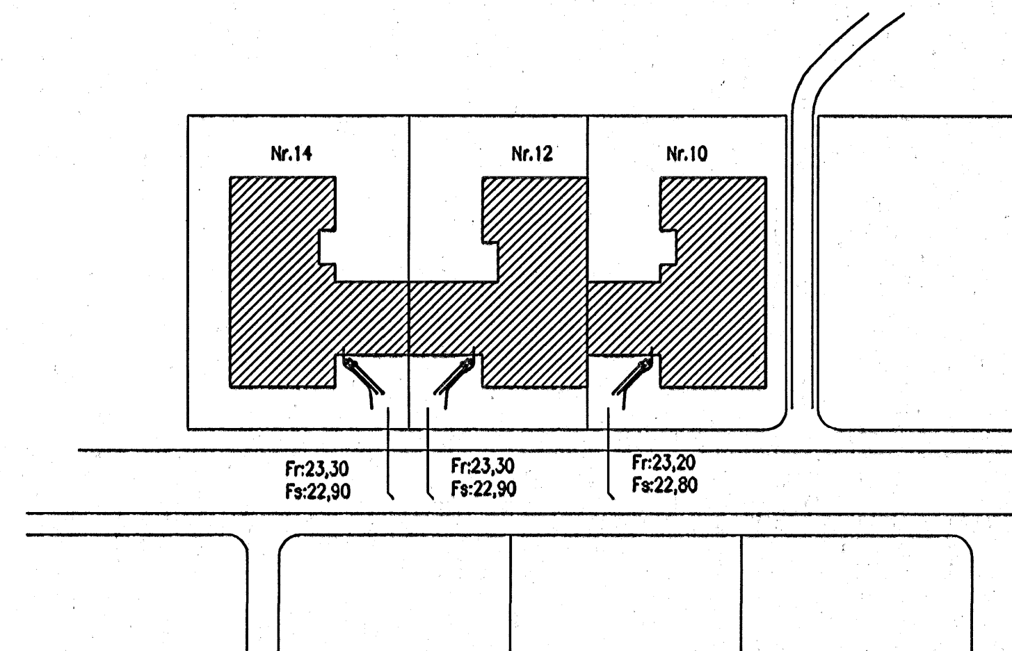
Afstöðumynd, 1:500
