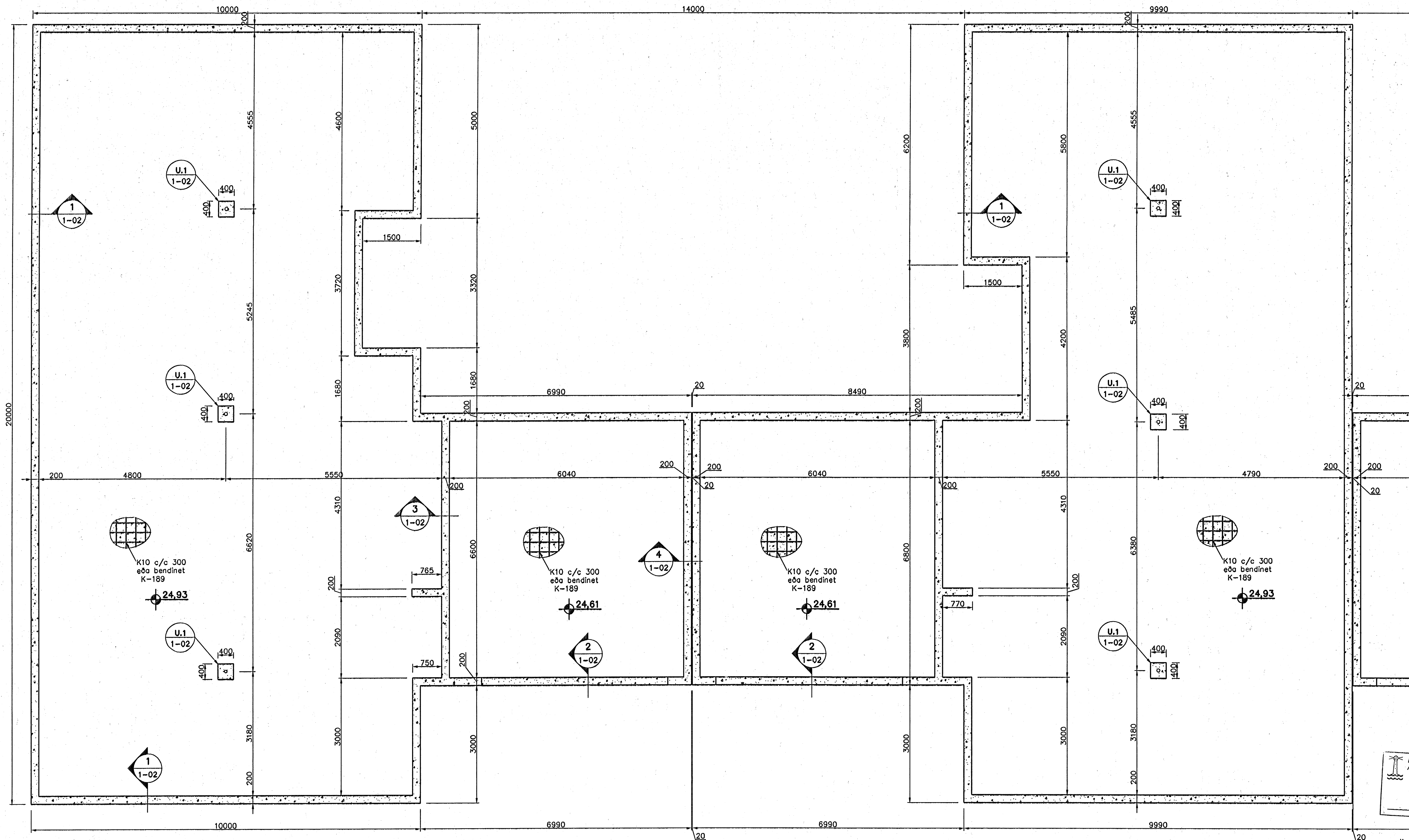
Undirstöður, Grunnmynd, 1:50
