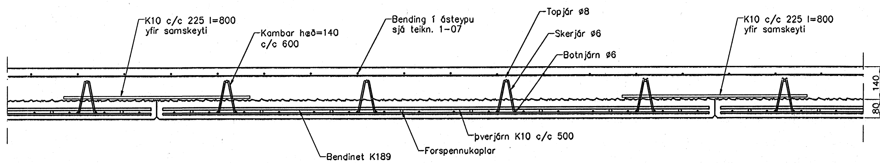
Filigranplötur, Sníð, 1:10
