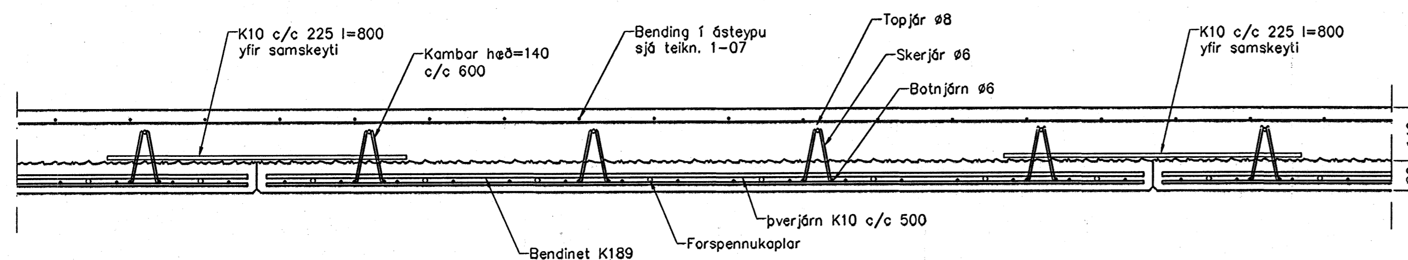
Filigranplötur, Snið, 1:10
