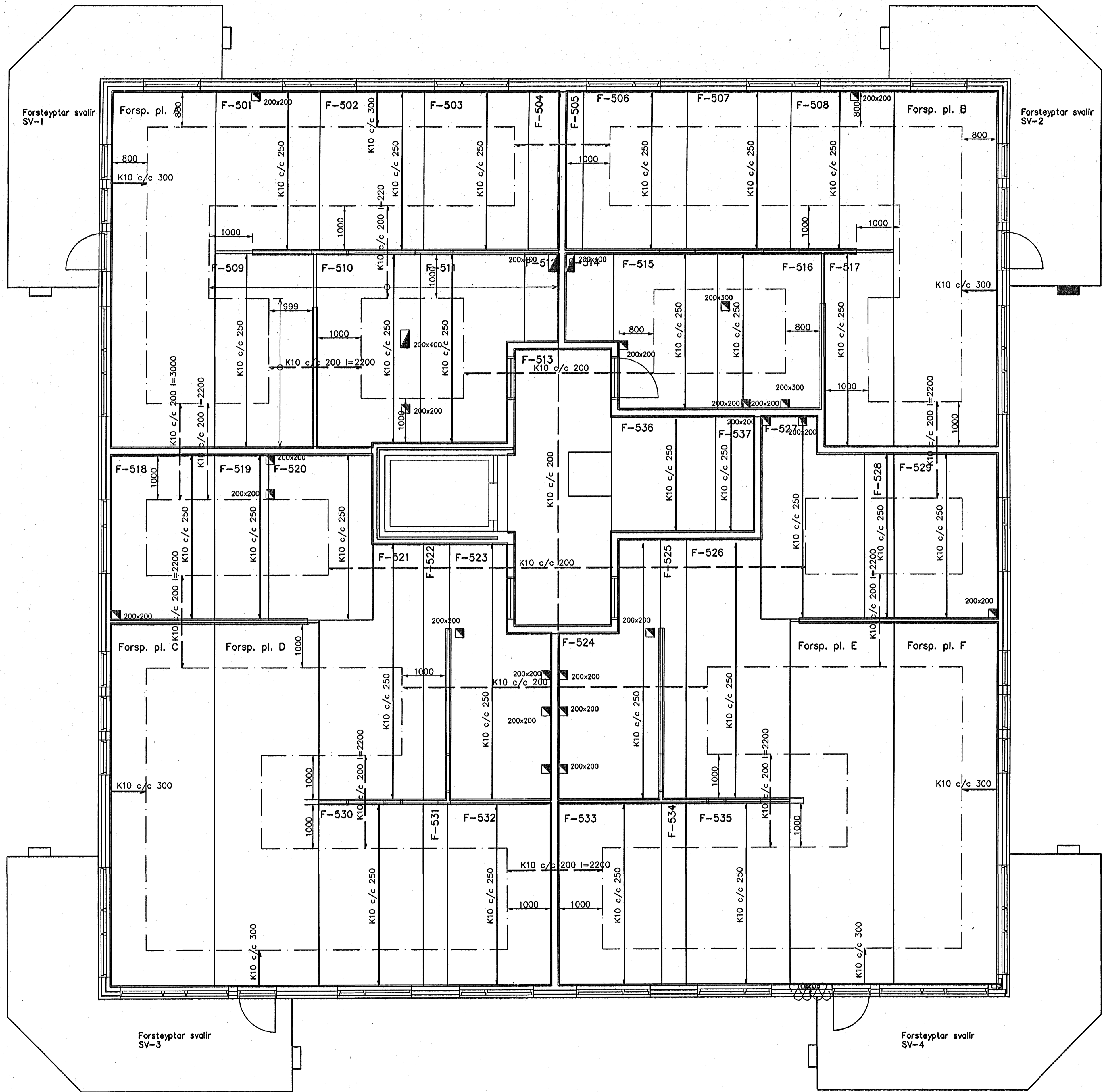
Plata yfir 1.hæð, Grunnmynd, 1:50
