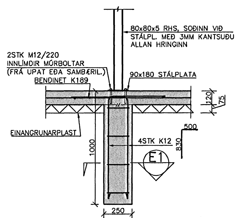
STÁLPLATA 1:5
