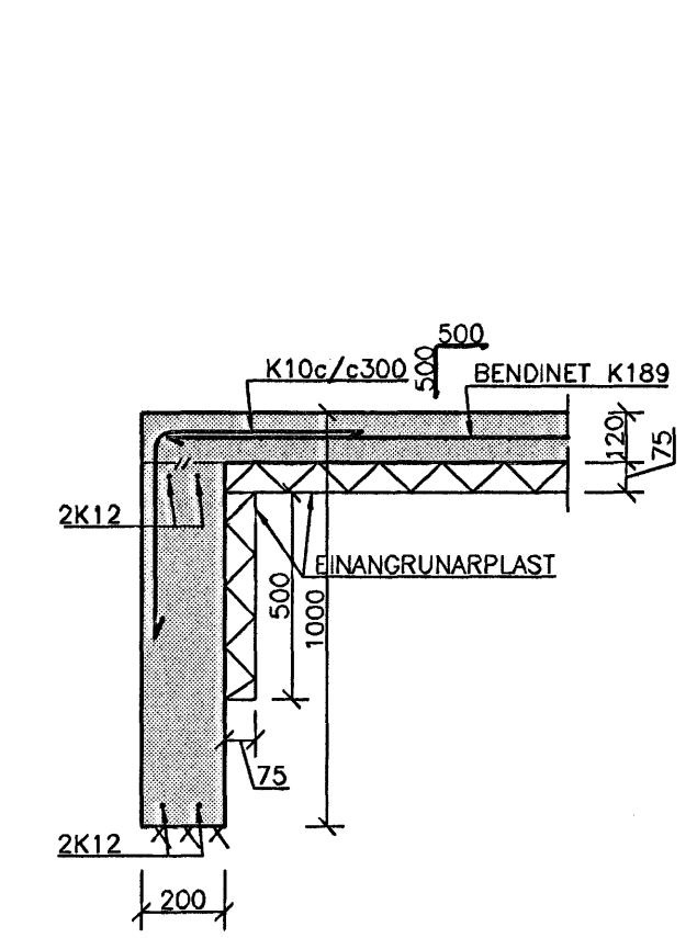
DEILI B 1:20
