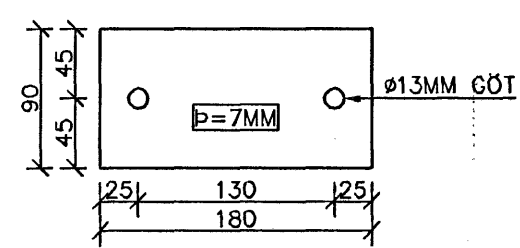
STÁLPLATA 1:5
