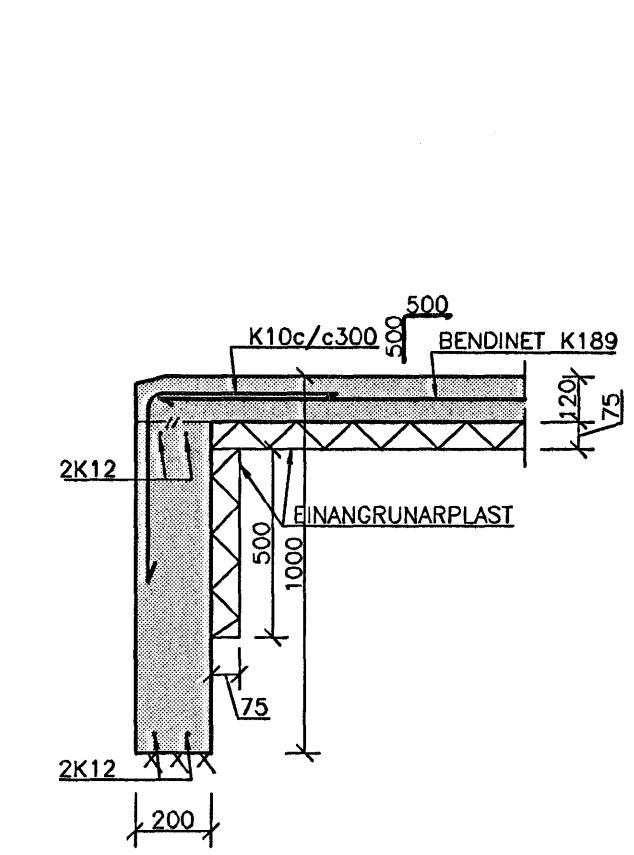
DEILI C 1:20
