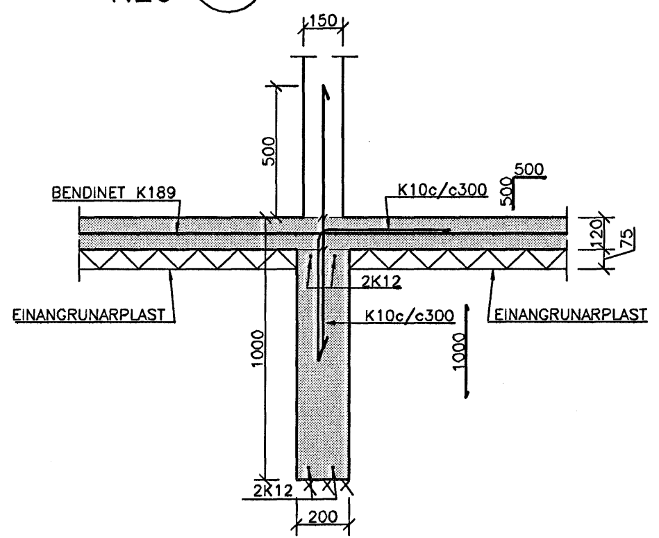
DEILI D 1:20
