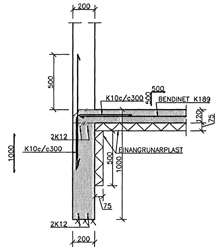
DEILI A 1:20
