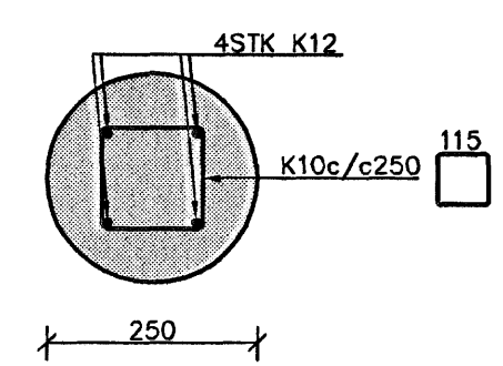
DEILI E1 1:10
