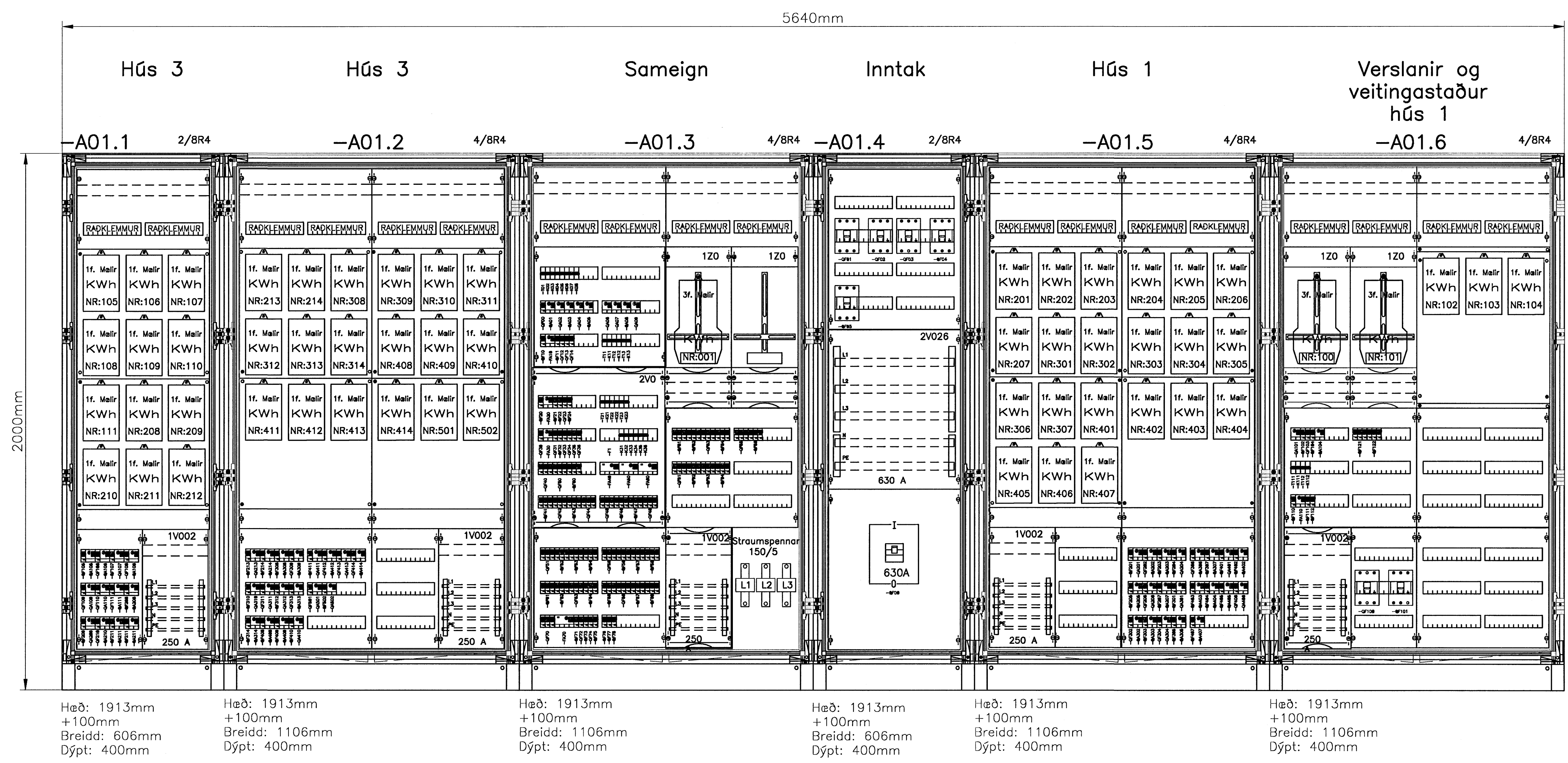
Aðaltafla -A01 Uppröðun búnaðar aðeins til viðmiðunar
