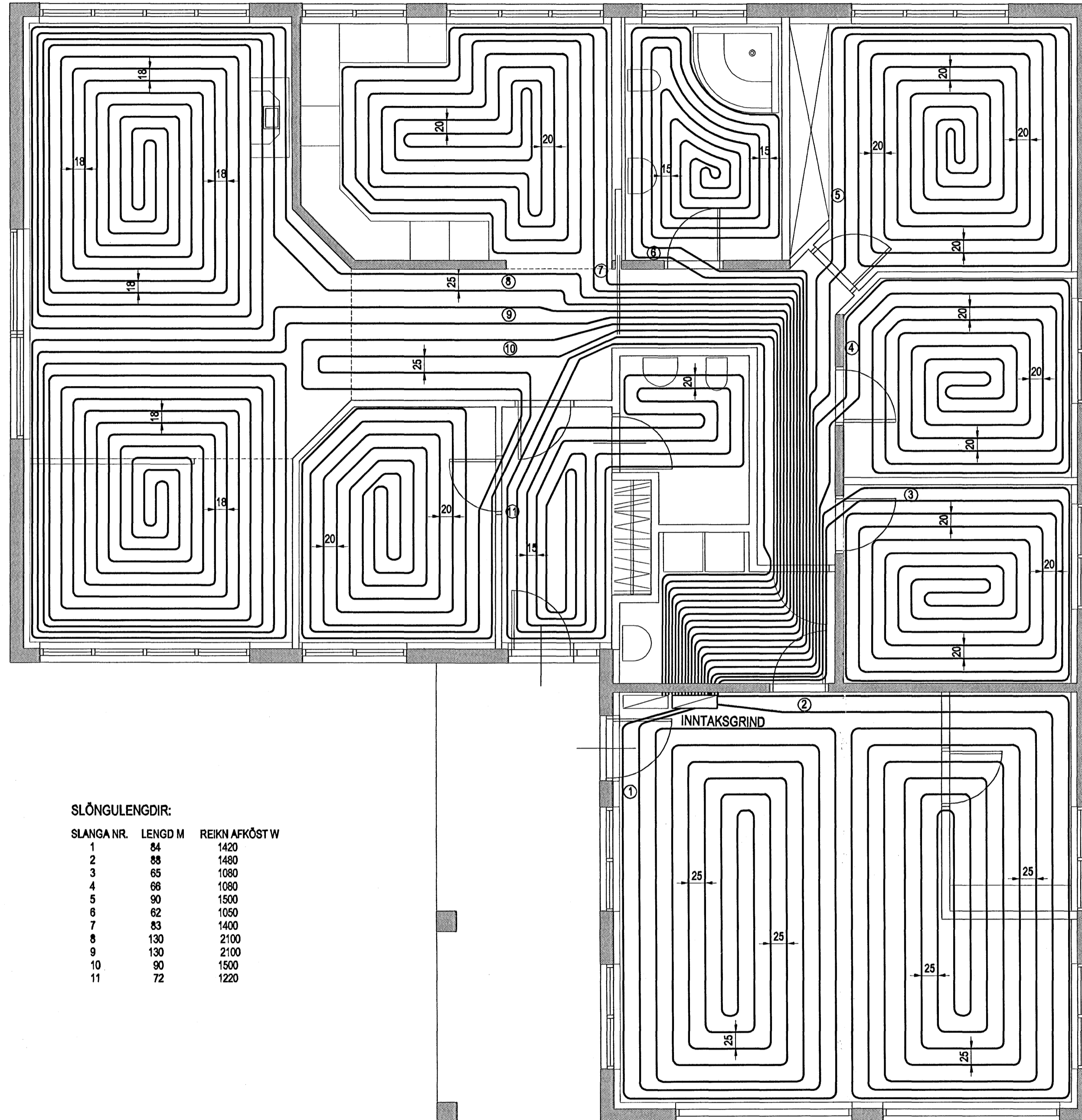
GÓLFHITALAGNIR - GRUNNMYND MKV. 1:50
