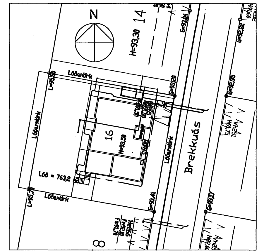
YFIRLITSMYND MKV. 1:500
