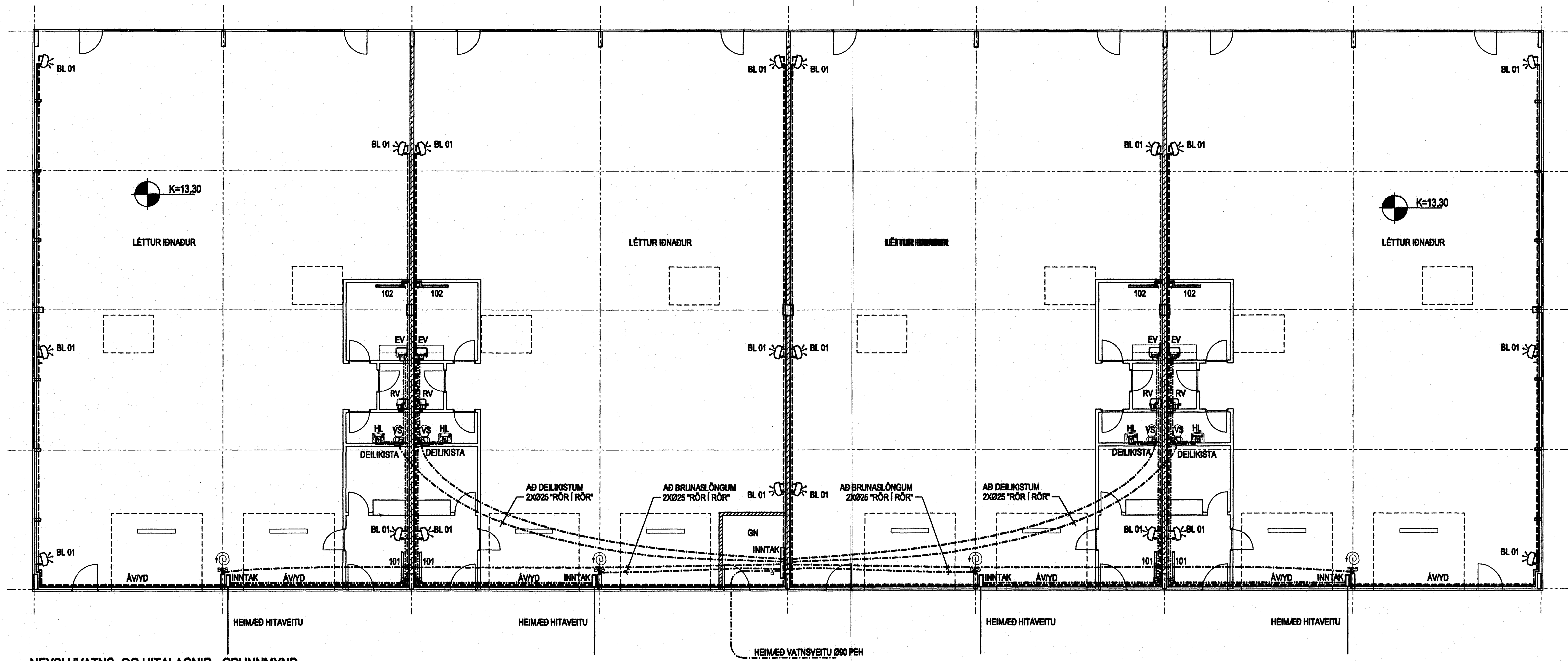
NEYSLUVATNS- OG HITALAGNIR - GRUNNMÝND MKV. 1:100
