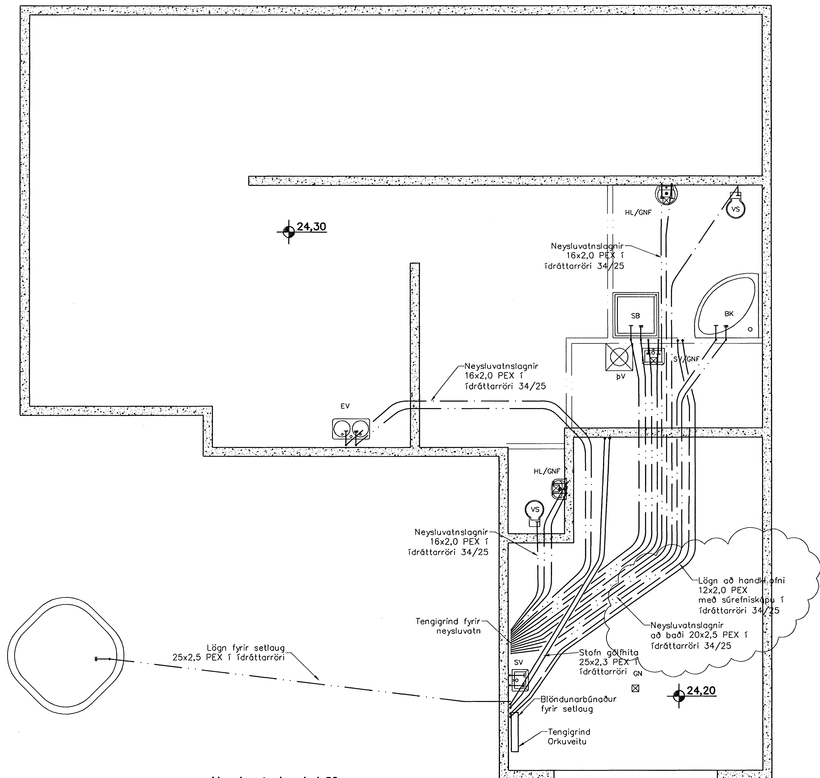
Neysluvatnslagnir 1:50
