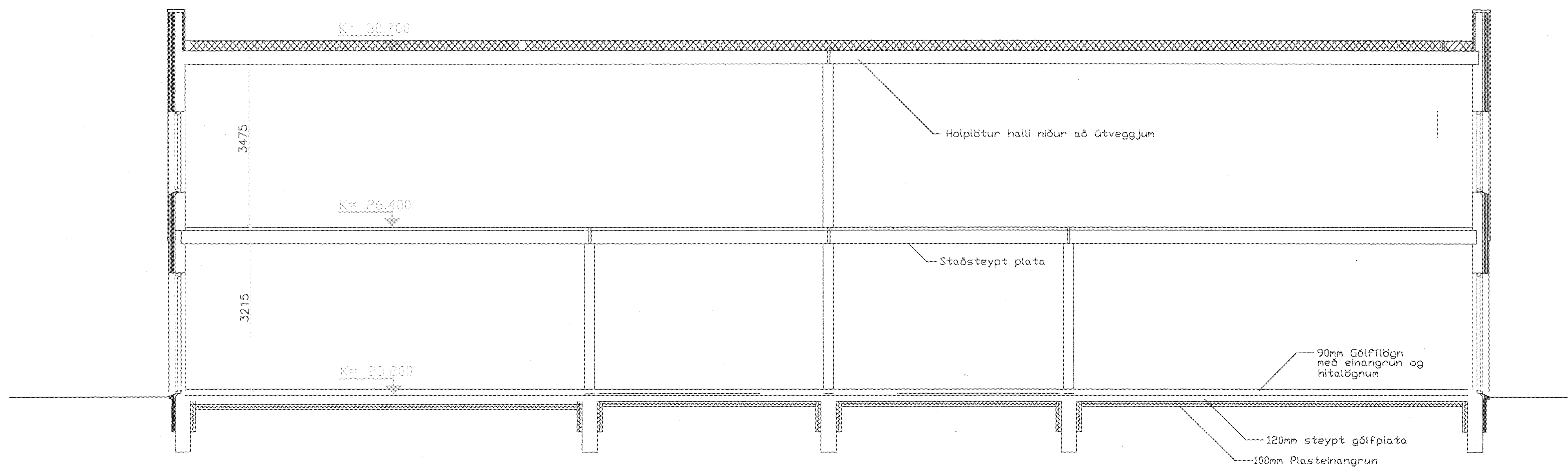
SNID G - G Mkv. 1: 50
