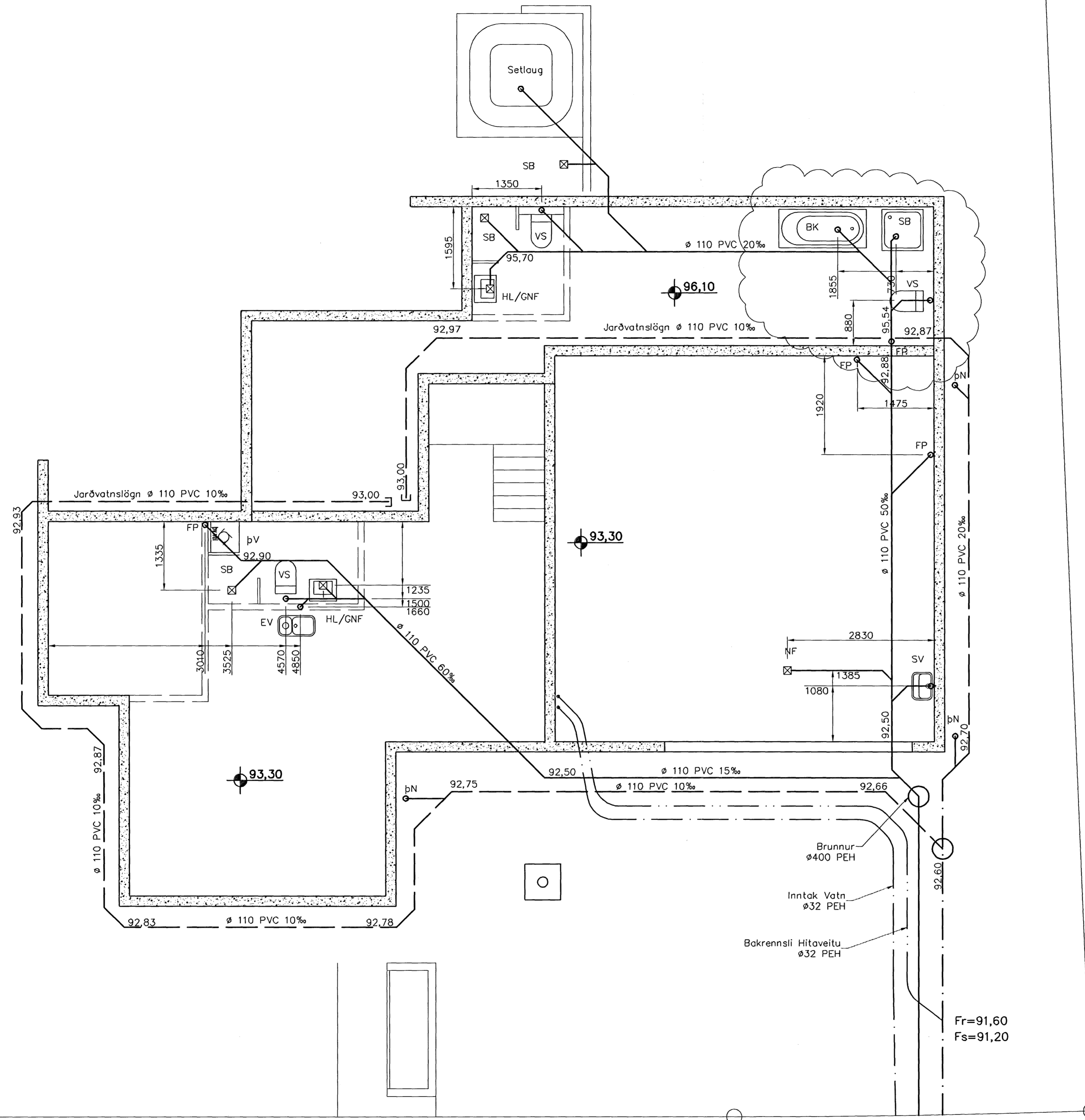
Grunnlagnir 1:50
