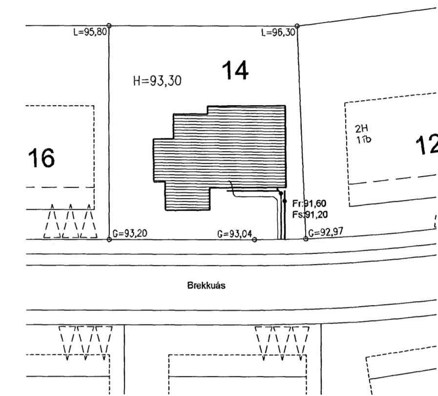
Afstöðumynd 1:500
