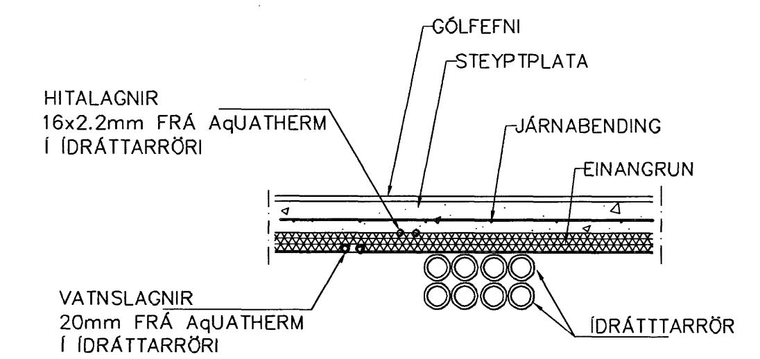
LAGNIR, SNIÐ, 1:20
