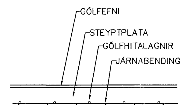
LAGNIR, SNIÐ, 1:20
