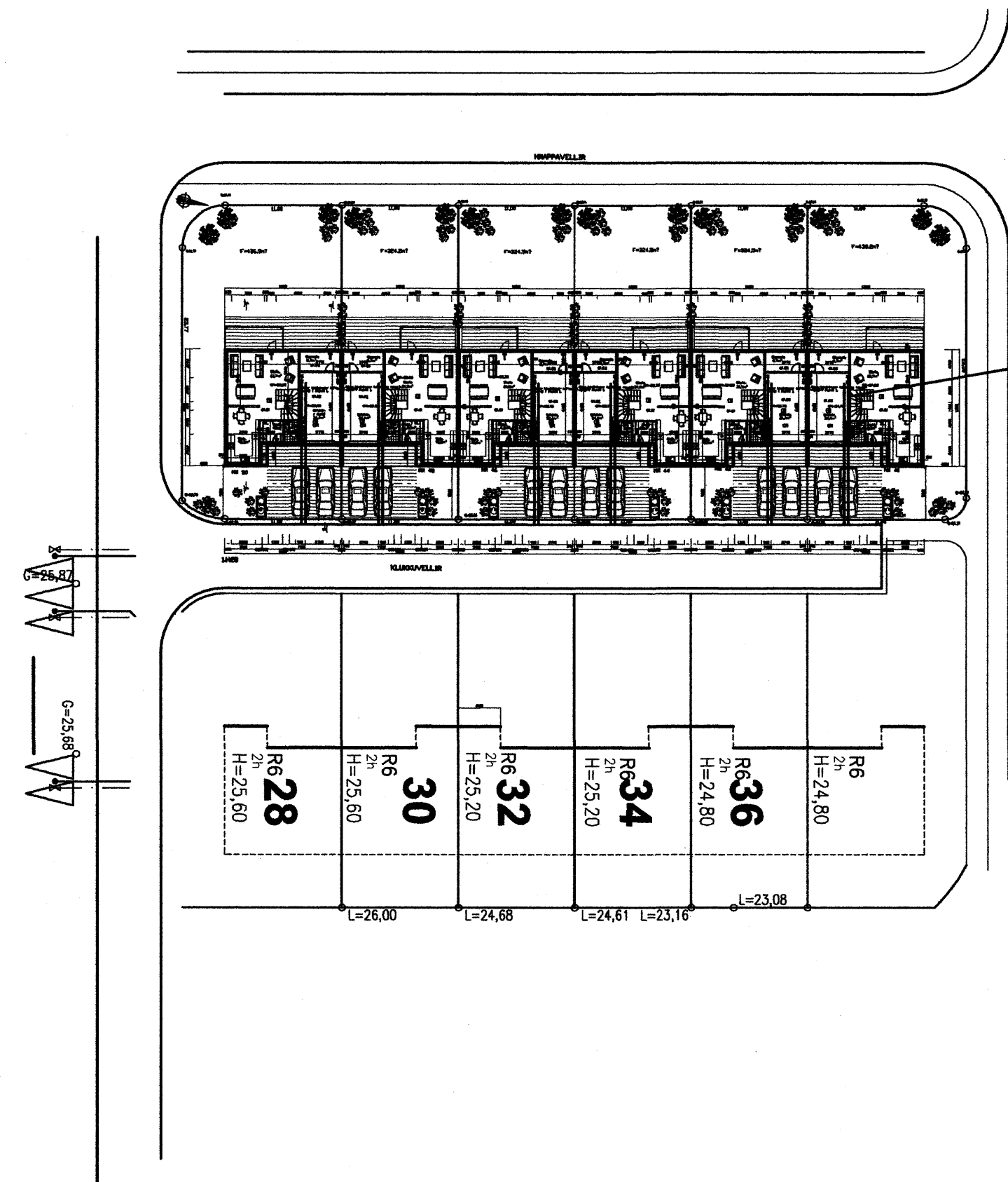
Afstöðmynd 1:500
