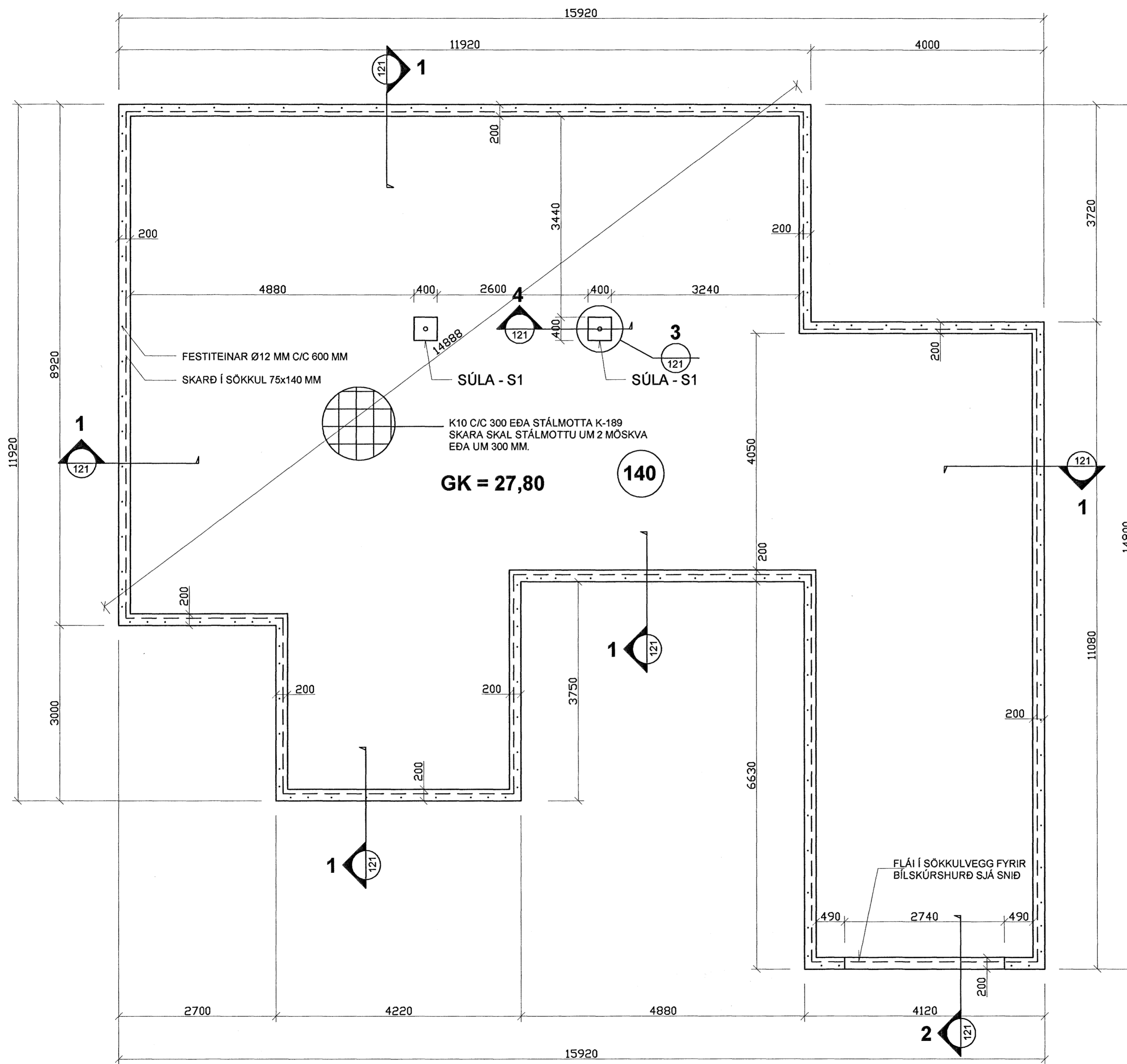
GRUNNMYND - 1:50
