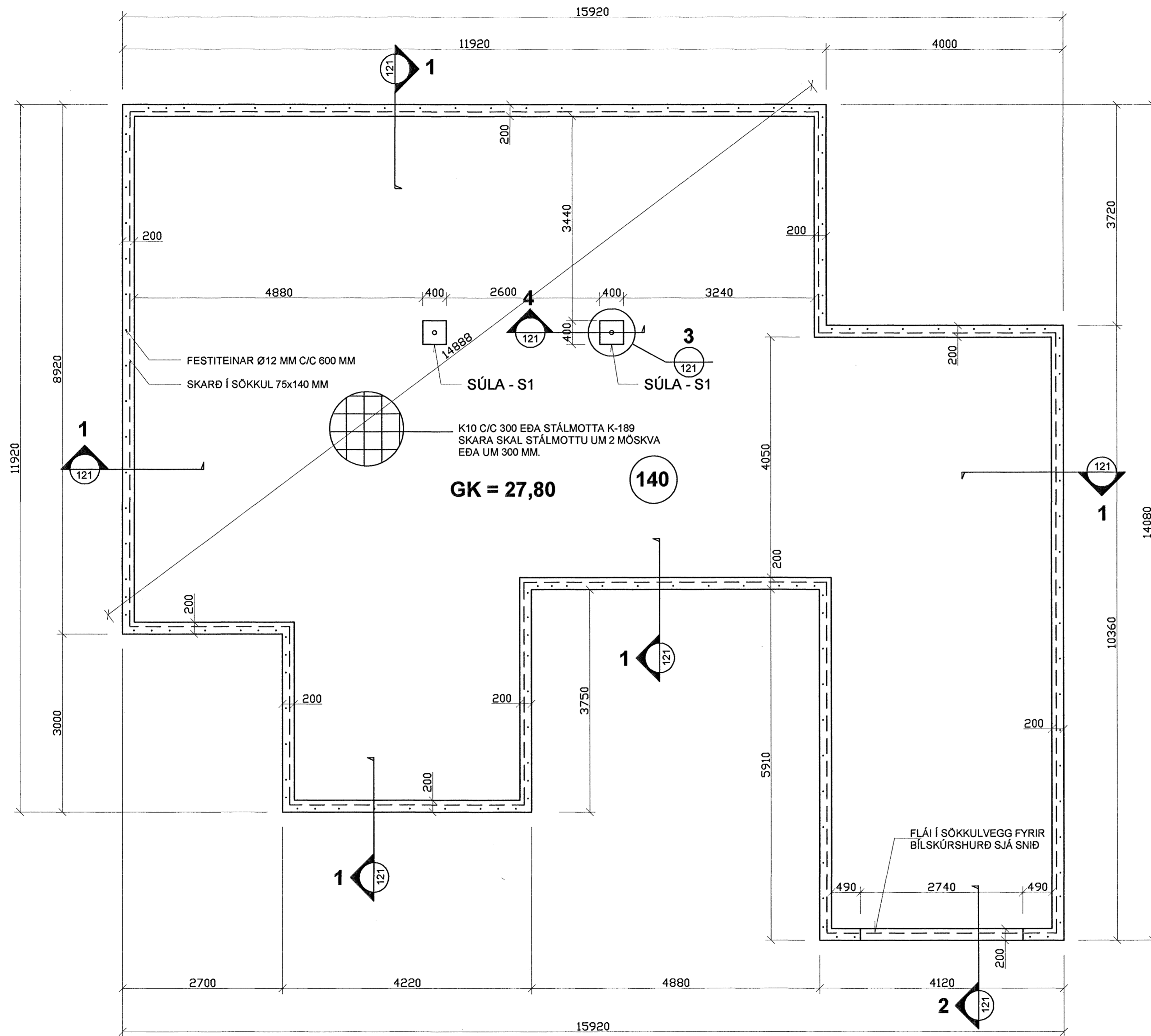
GRUNNMYND - 1:50
