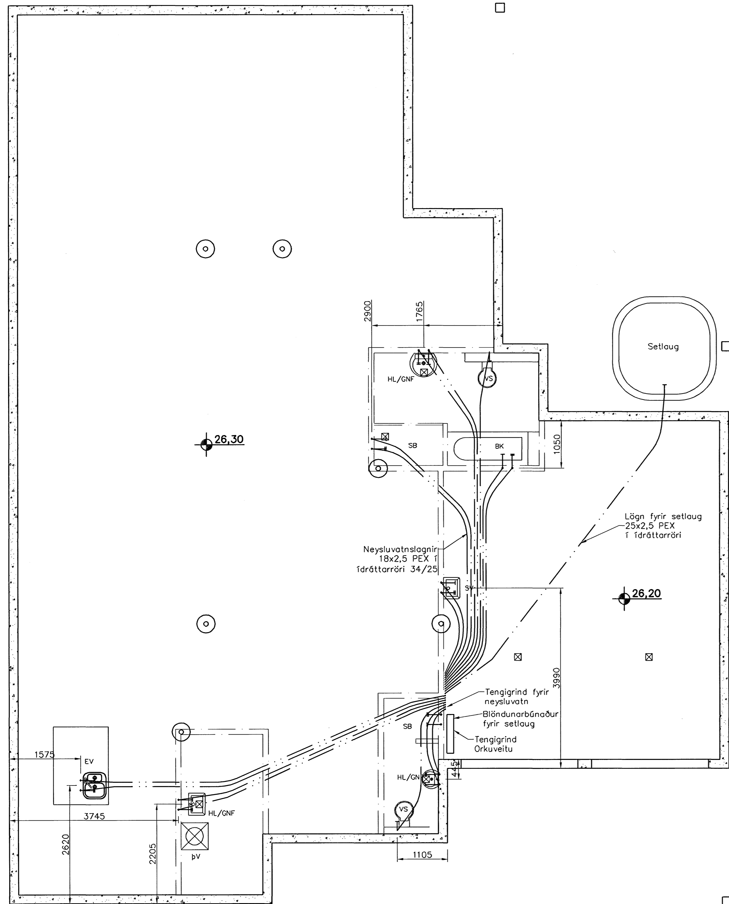
Neysluvatnslagnir 1:50
