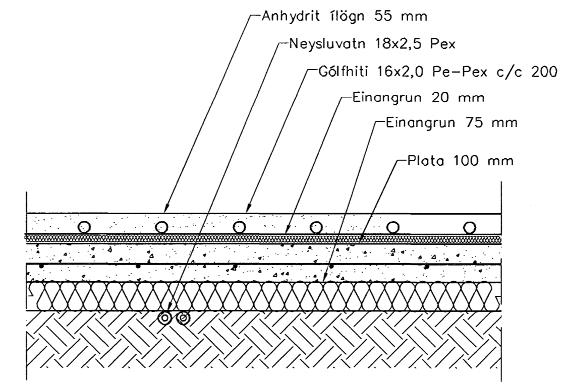
Hita- og vatnslagnir, Snið í botnplötu, 1búð 1:10
