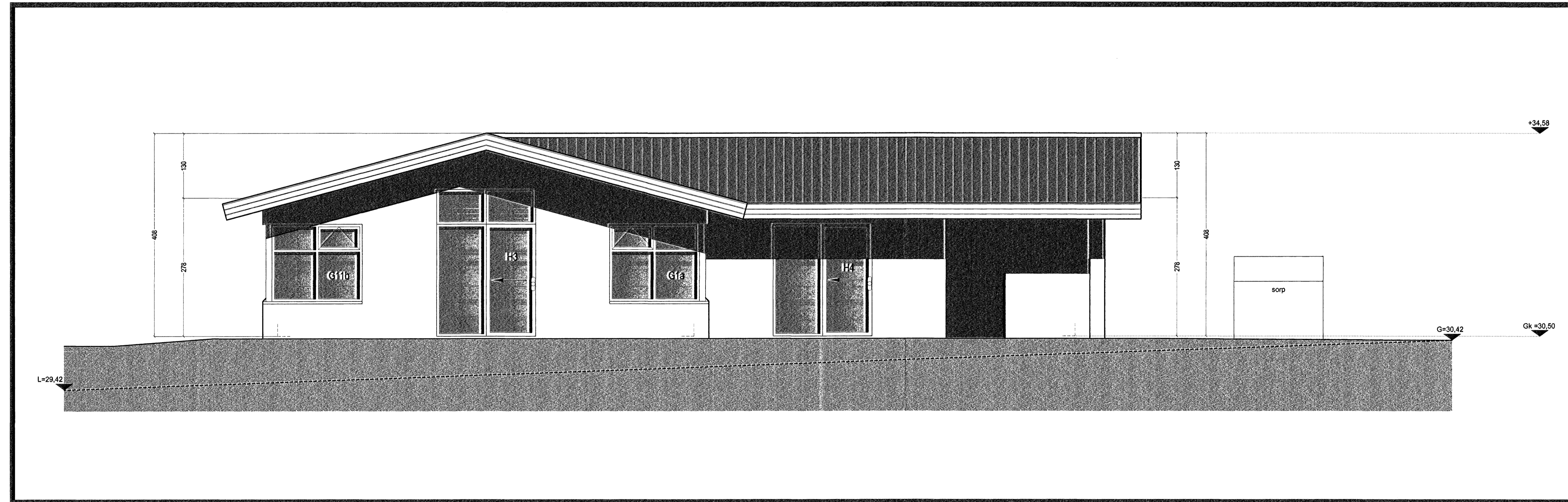
Vestur útlit 1:50
