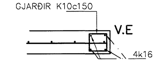
VEGGDAR 1:20
