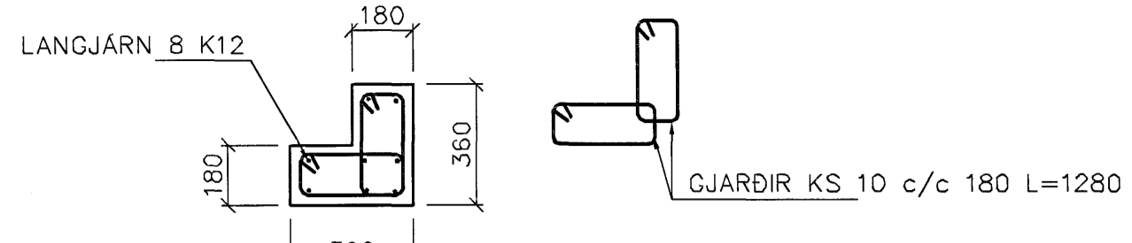
SÓLA S2 1:20
