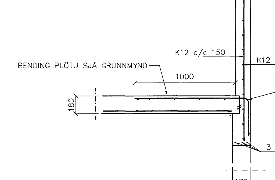
SNID 6 1:20
