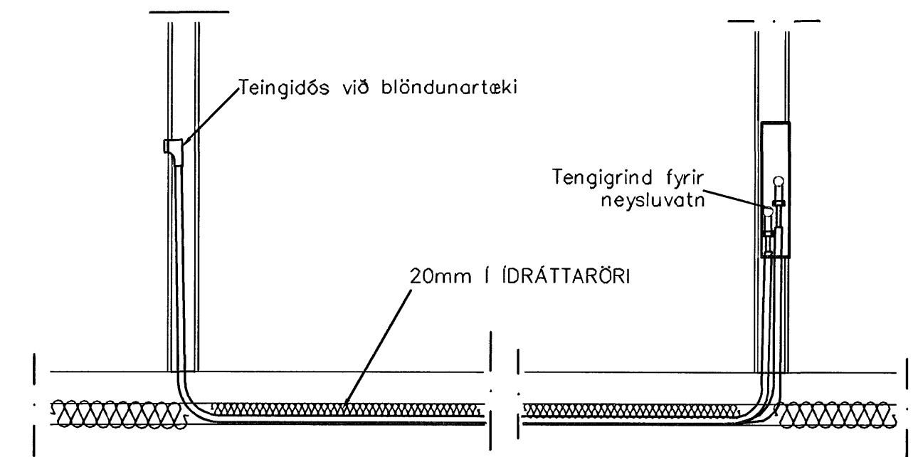
LAGNIR, SNIÐ, 1:20
