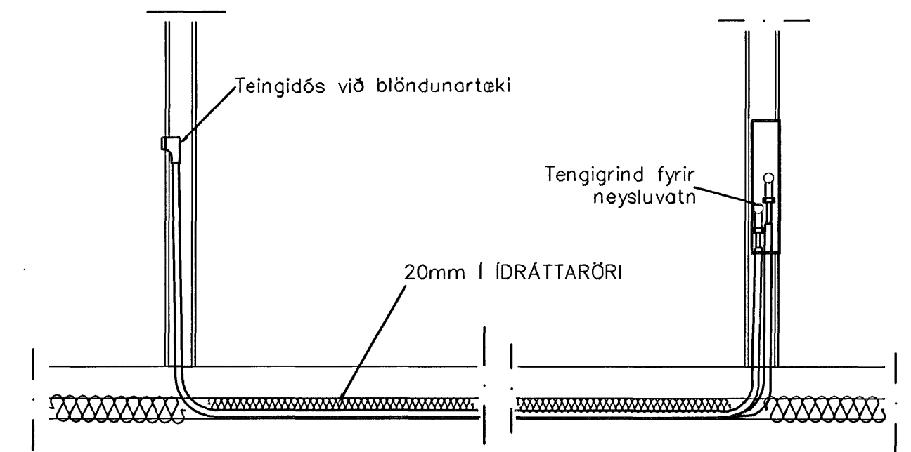
TENING NEYSLUVATNSLAGNA 1:20
