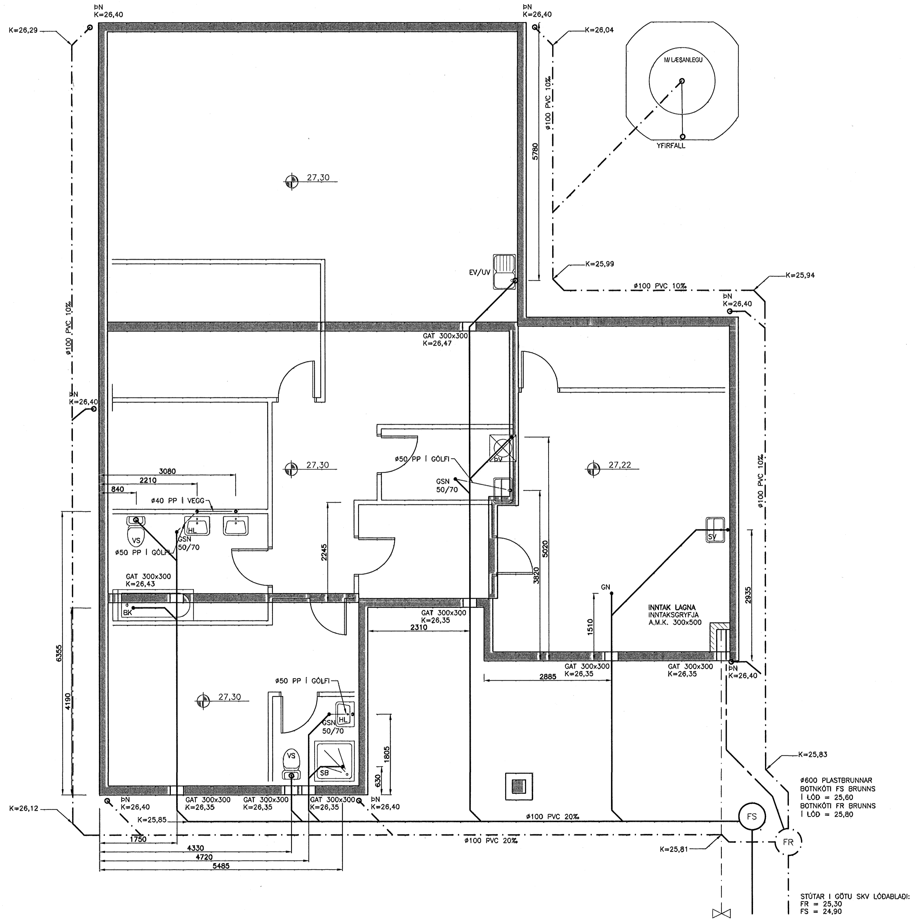
GRUNNMYND FRÄRENNISLAGNA Mkv. 1:50
